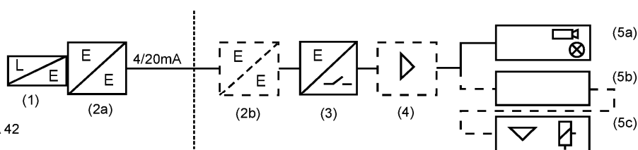
Schema der Leckagesonde für alle Typen und eingebautem Messumformer FEL60H
