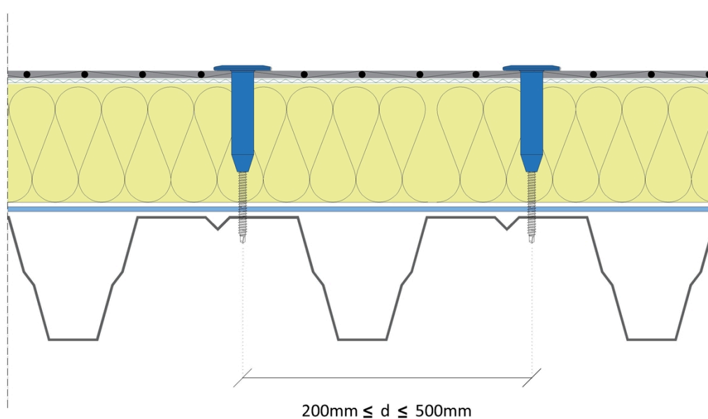
Abbildung A5-2: Minimaler und maximaler Abstand zwischen den Befestigern (in Längsrichtung zum Kunststoffprofil)
