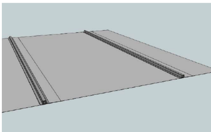
Abbildung A1-2: Dachabdichtungsbahn mit aufgeschweißten Kunststoffprofilen
