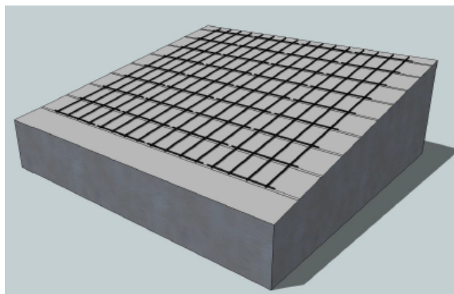
Abbildung A1-3: Überblick über das Gesamtsystem einschließlich Unterkonstruktion der Solaranlage
