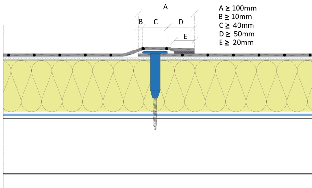
Abbildung A2-1: Überlappungsstoß der Naht
