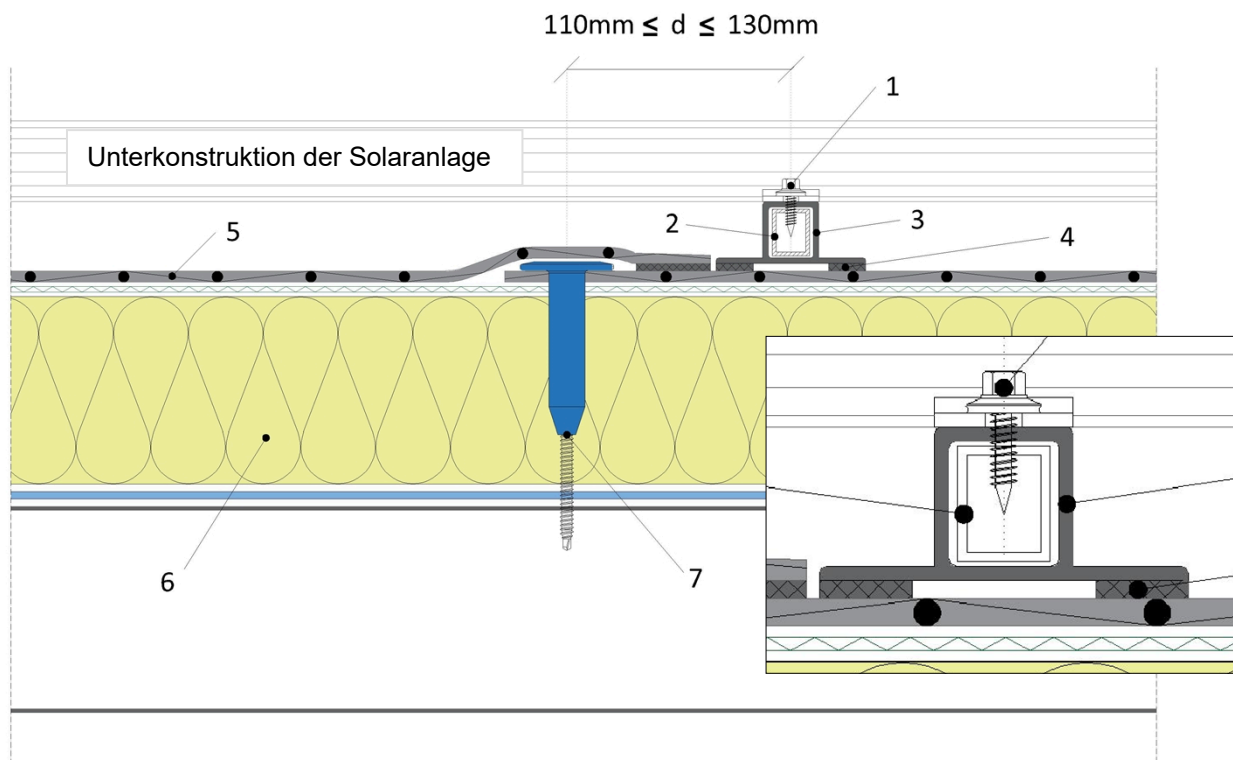
Abbildung A1-1: Querschnitt
