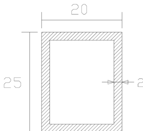
Abbildung A3-1: Aluminiumprofil "RENOLIT ALKORPLUS 81601"
