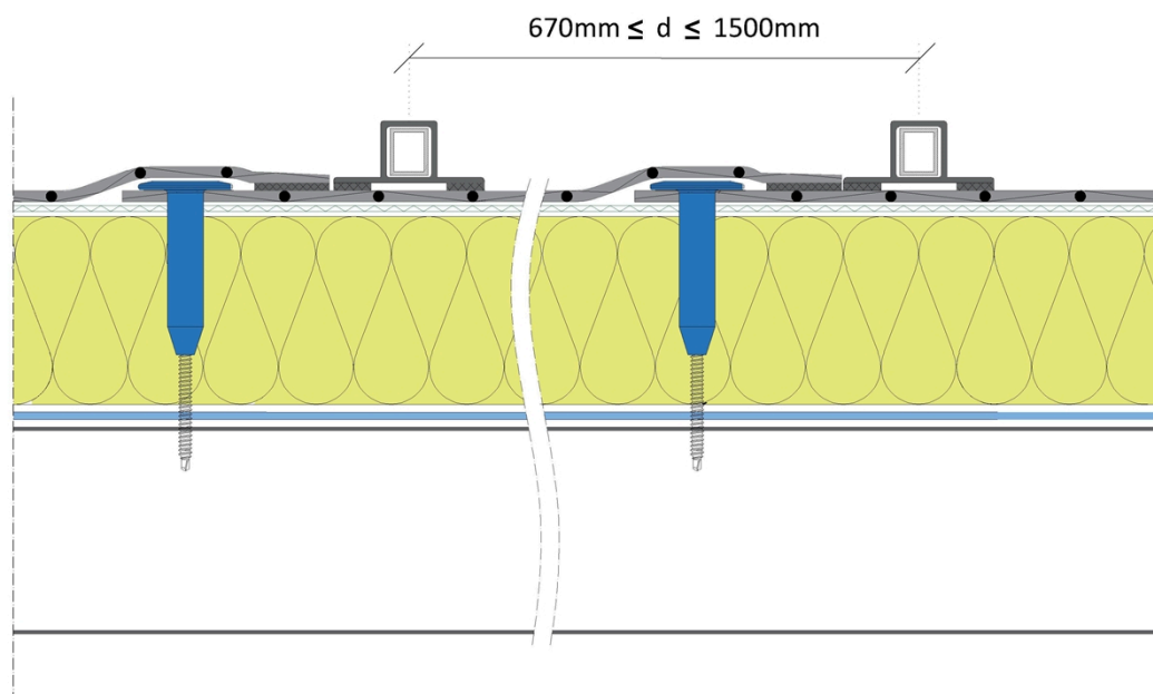
Abbildung A5-1: Minimaler und maximaler Abstand zwischen den Kunststoffprofilen
