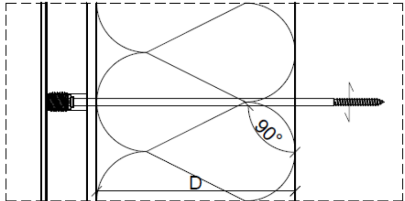
Detail horizontale Verschraubung (Ansicht)
