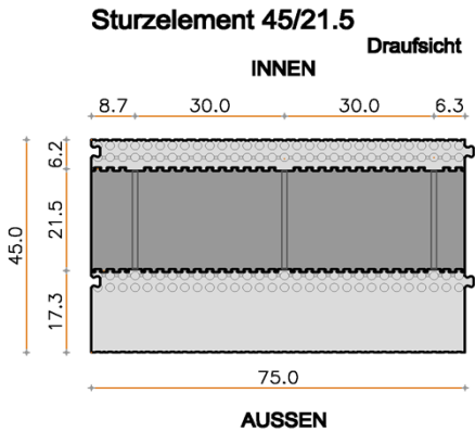
Abmessungen Sturzelement 45/21.5 (75x45x30)
