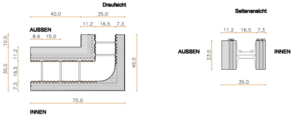
Abmessungen Eckelement Innen 35/16.5 (45-75)x35x23
