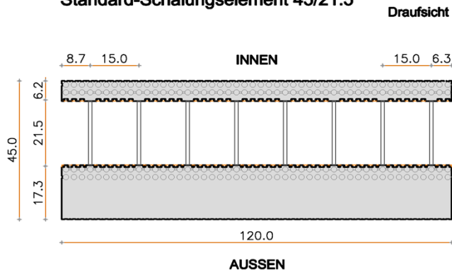
Abmessungen Standard-Schalungselement 45/21.5 (120x45x30)
