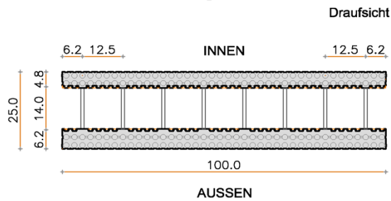
Abmessungen Standard-Schalungselement 25/14.0 (100x25x25)
