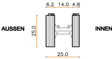
Seitenansicht
