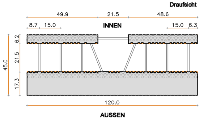
Abmessungen "T"-Element 45/21.5 (120x45x30)
