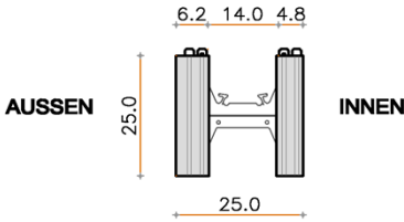
Seitenansicht
