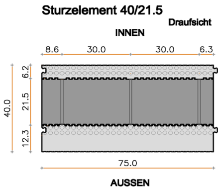
Abmessungen Sturzelement 40/21.5 (75x40x30)
