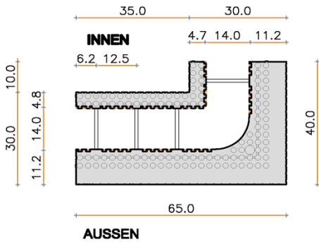
Abmessungen Eckelement 30/14.0 (65-40)x30x25
