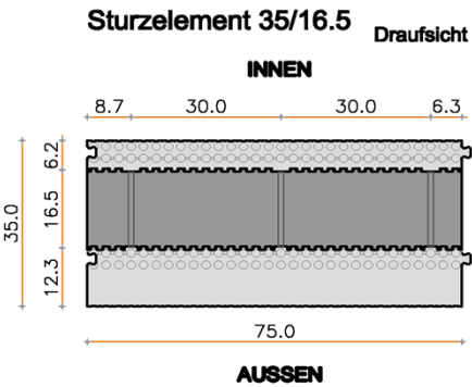
Abmessungen Sturzelement 35/16.5 (75x35x30)
