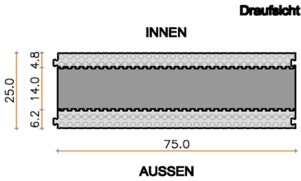
Abmessungen Sturzelement 25/14.0 (75x25x25)
