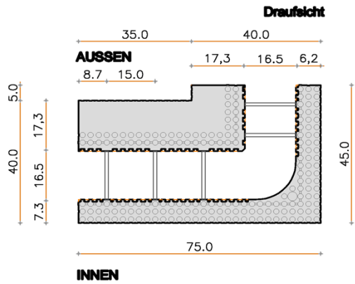
Abmessungen Eckelement Innen 40/16.5 (45-75) 40x30
