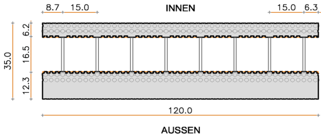
Abmessungen Standard-Schalungselement 35/16.5 (120x35x30)
