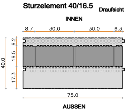
Abmessungen Sturzelement 40/16.5 (75x40x30)
