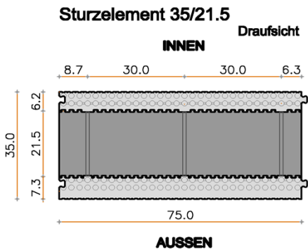
Abmessungen Sturzelement 35/21.5 (75x35x30)
