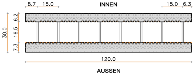
Abmessungen Standard-Schalungselement 30/16.5 (120x30x30)
