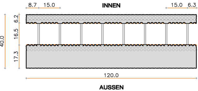
Abmessungen Standard-Schalungselement 40/16.5 (120x40x30)
