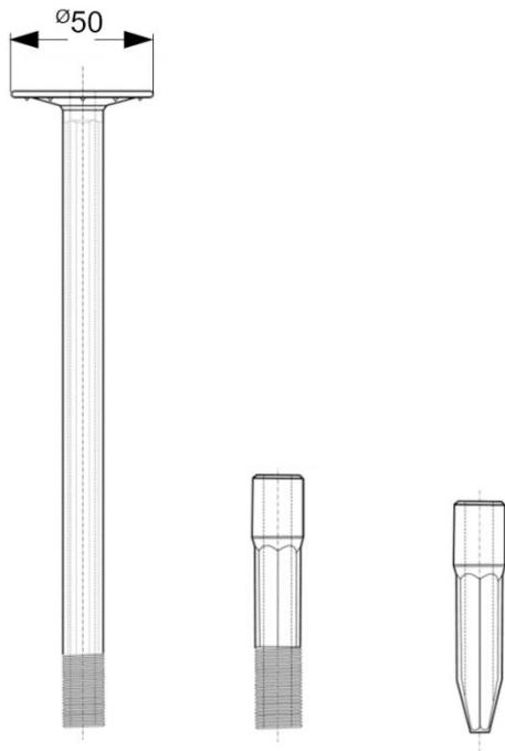
Zahn ZKSH round module 4,8
