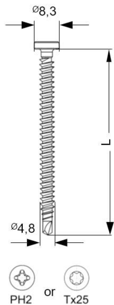
Zahn ZDBK-E 4,8 x L
