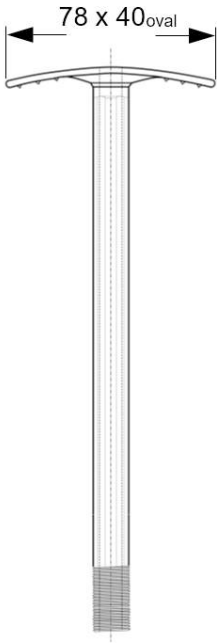
Zahn ZKSH oval module 4,8
