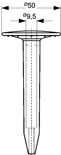
Zahn ZKSH gray / round
