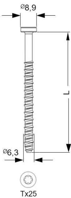
Zahn ZBST 6,3 x L
