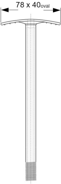
Zahn ZKSH oval module 4,8
