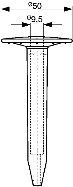
Zahn ZKSH round
