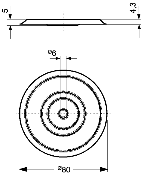
Zahn ZCTS 1 -plate
