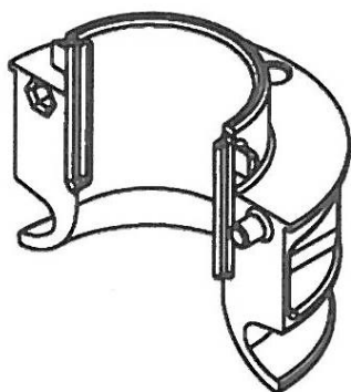
"Montagehülse"
