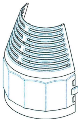
"Dichtdeckel", Halbschale
