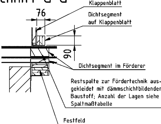
Schnitt G-G
