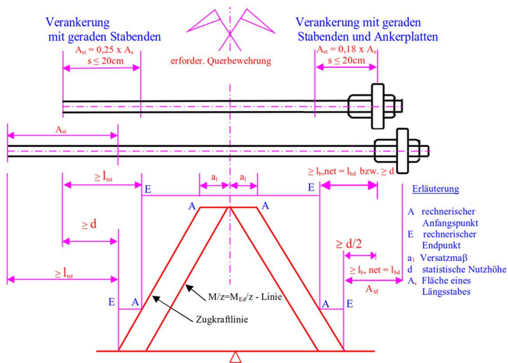
Bild 3b Beispiel für die Verankerung von Stäben \varnothing 40 bzw. 50 mm mit geraden Stabenden und Ankerplatten im Stützbereich massiger Bauteile
