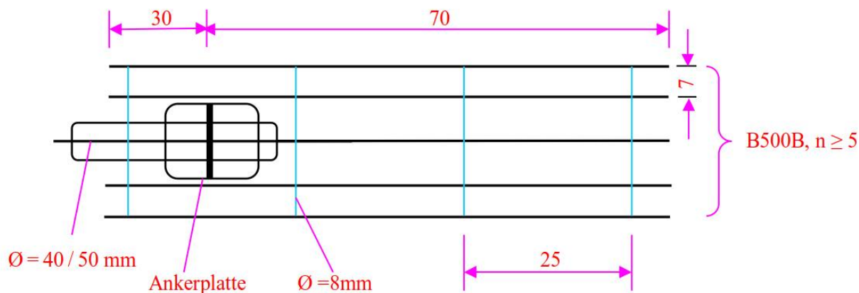
Beispiel für die Rückverankerung von Ankerplatten
