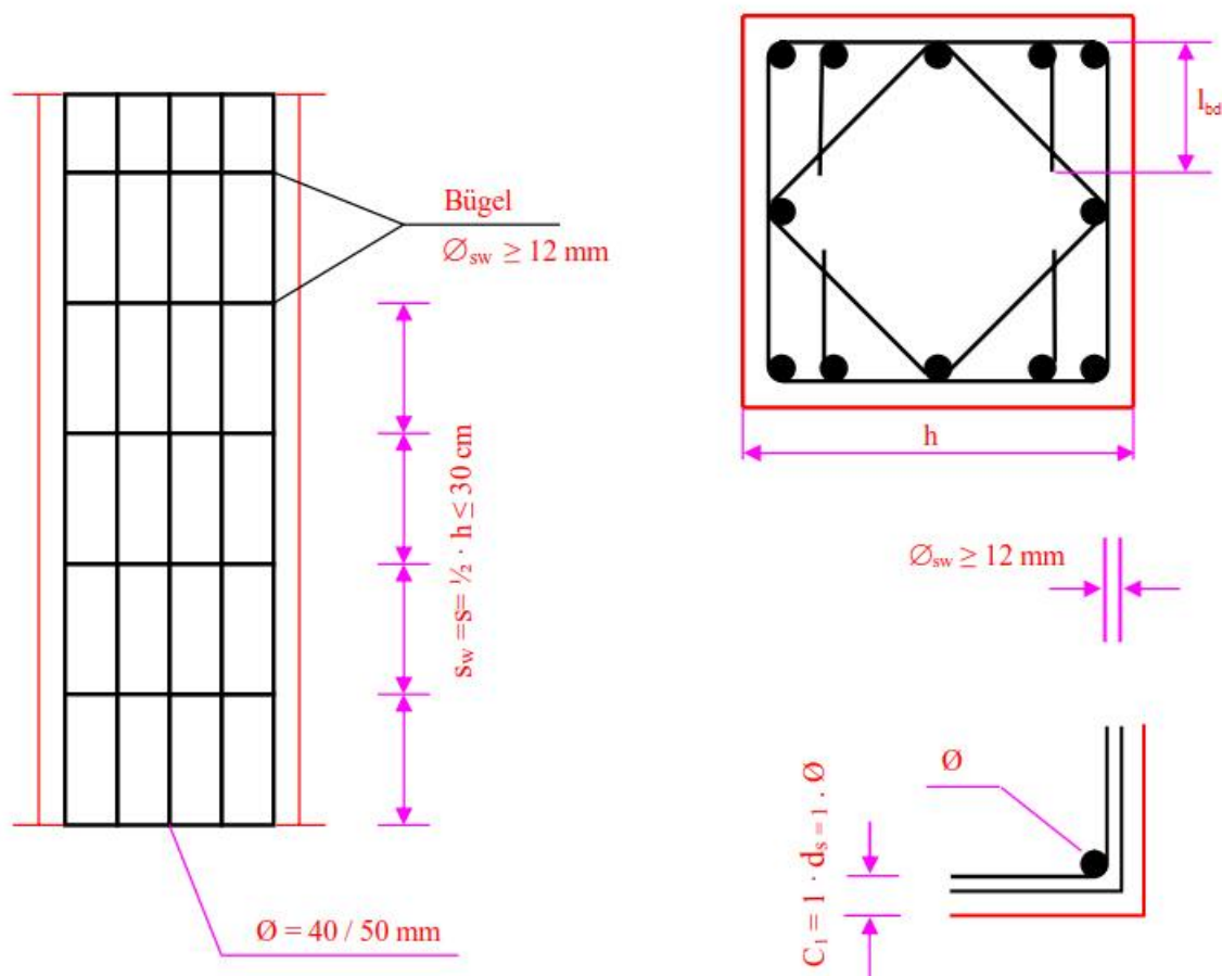
Beispiel für die Bewehrung einer Stütze
