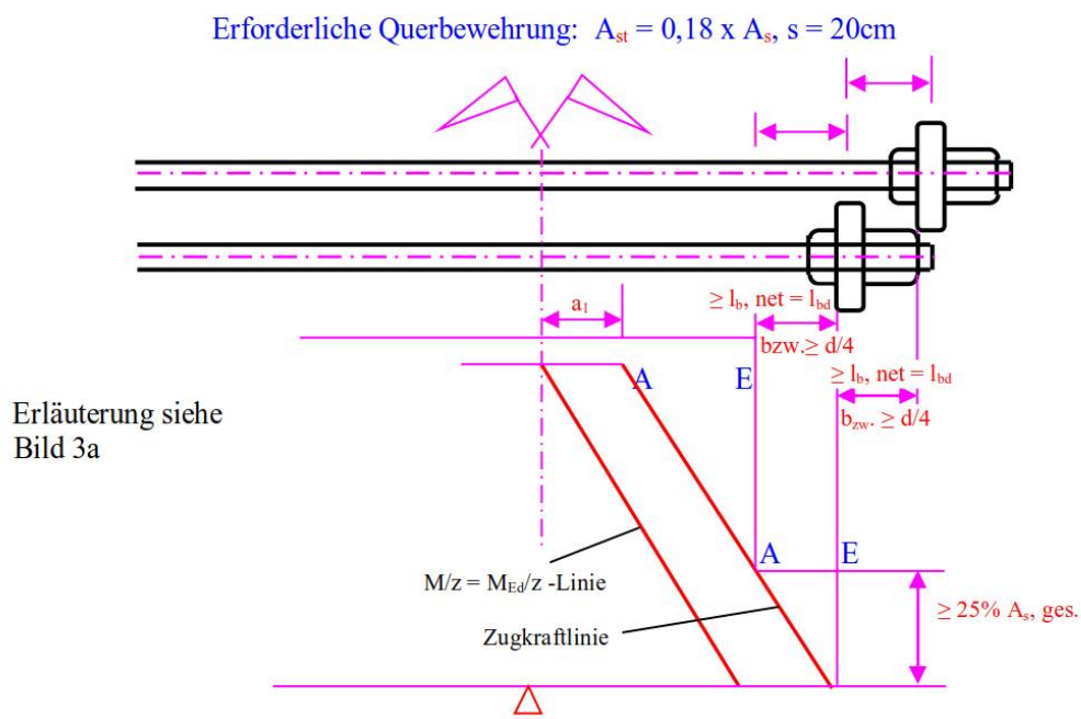
Bild 3b Beispiel für die Verankerung von Stäben \varnothing 40 bzw. 50 mm mit geraden Stabenden und Ankerplatten im Stützbereich massiger Bauteile
