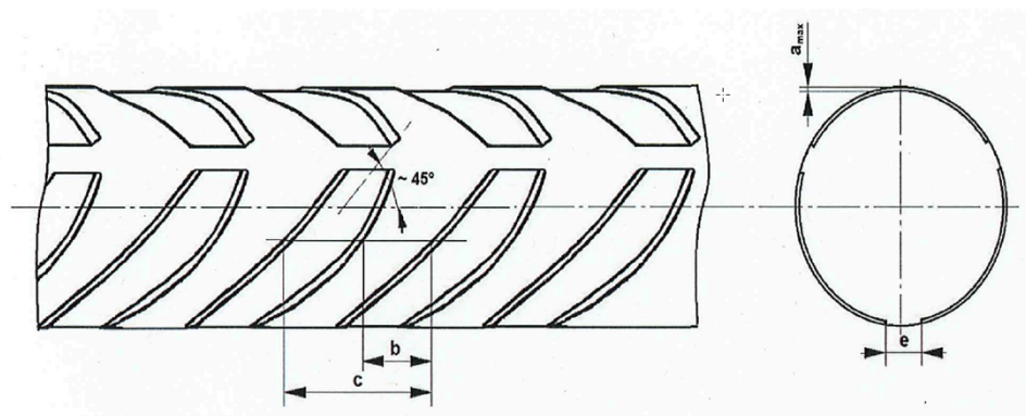
Bild 1: Ansicht des sonderprofilierten Spannstahls
