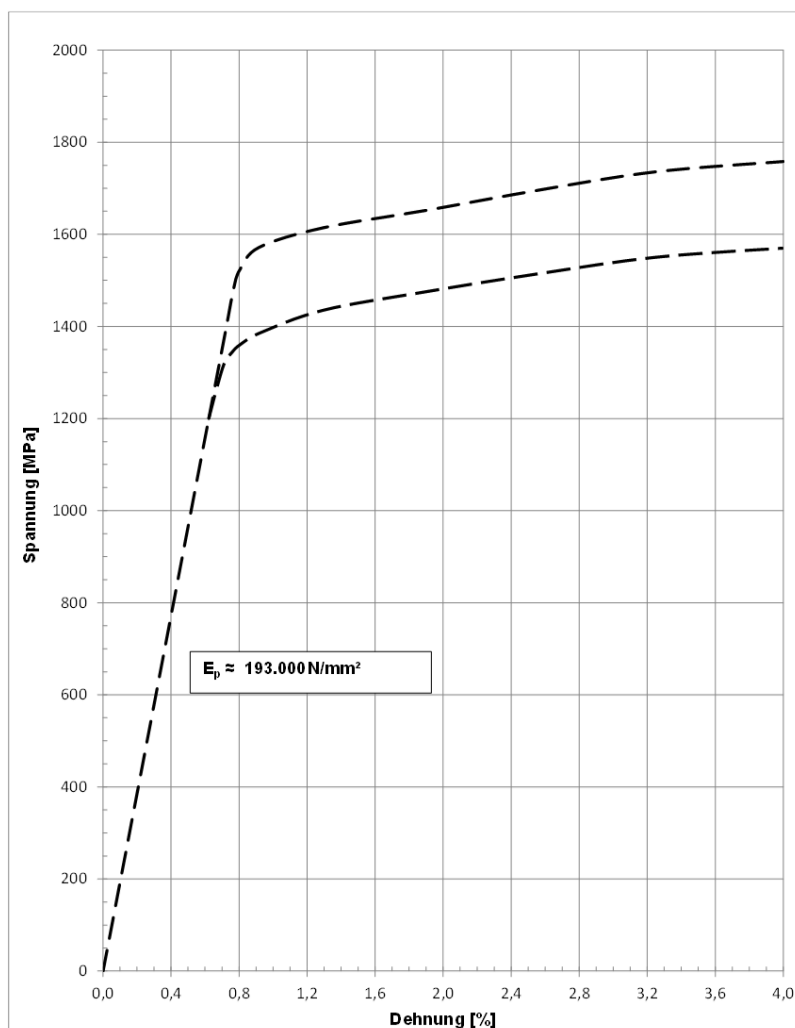
Bild 2: Prinzipieller Spannungs-Dehnungs-Verlauf
