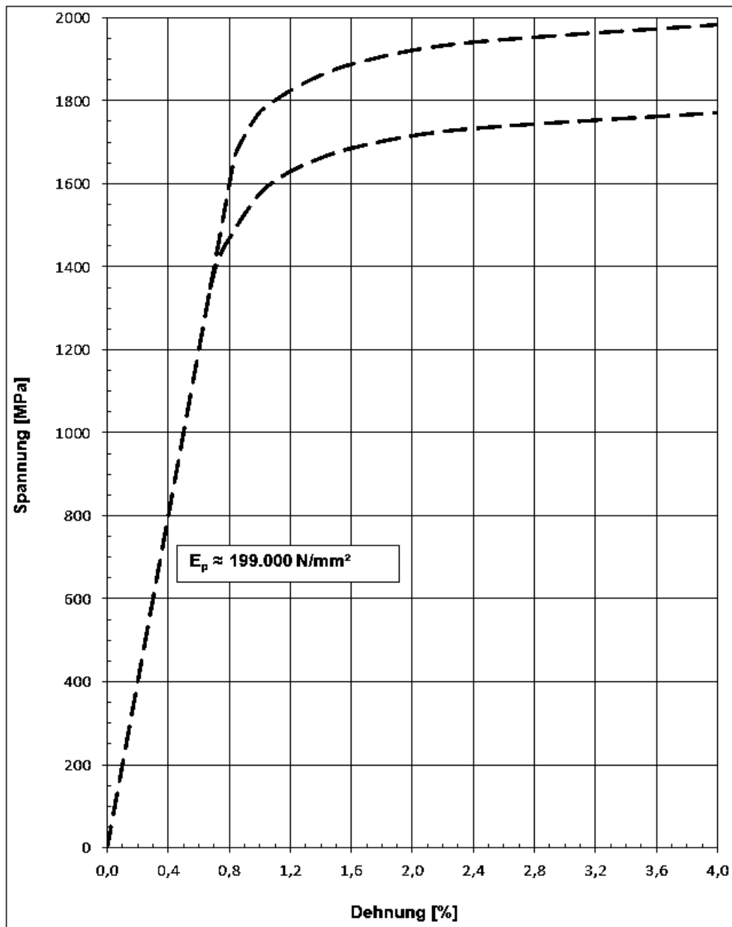
Bild 2: Prinzipieller Spannung-Dehnungs-Verlauf
