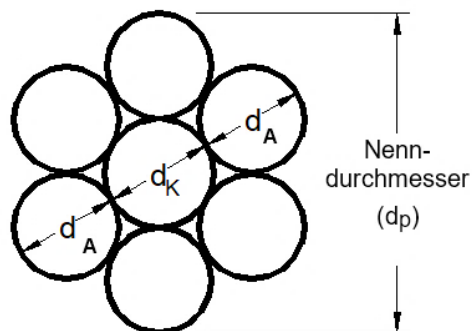
Bild 1: Darstellung des Spannstahlitzen-Querschnitts
