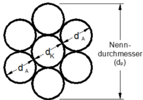
Bild 1: Darstellung des Spannstahllitzen-Querschnitts
