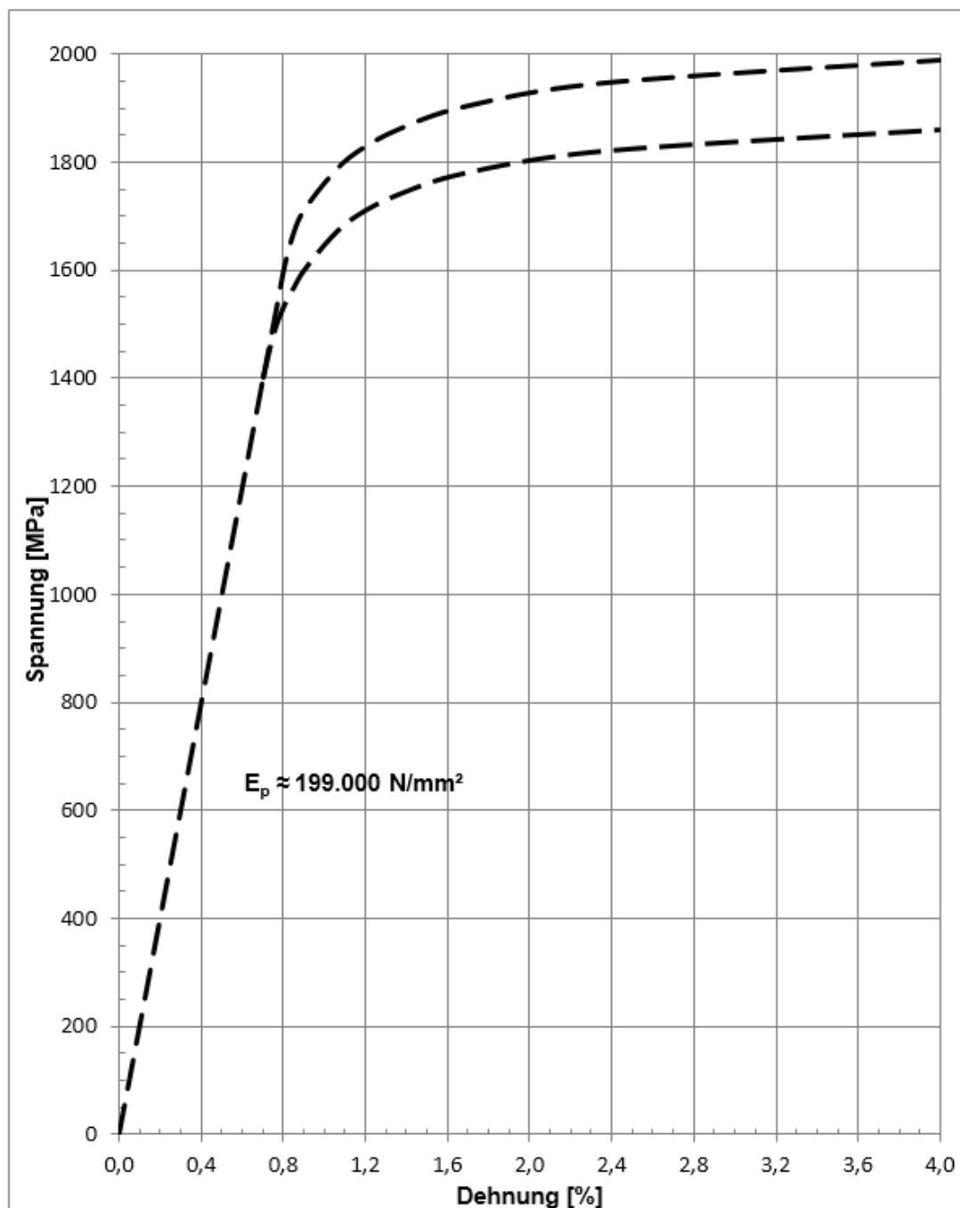
Bild 2: Prinzipieller Spannungs-Dehnungs-Linie-Verlauf
