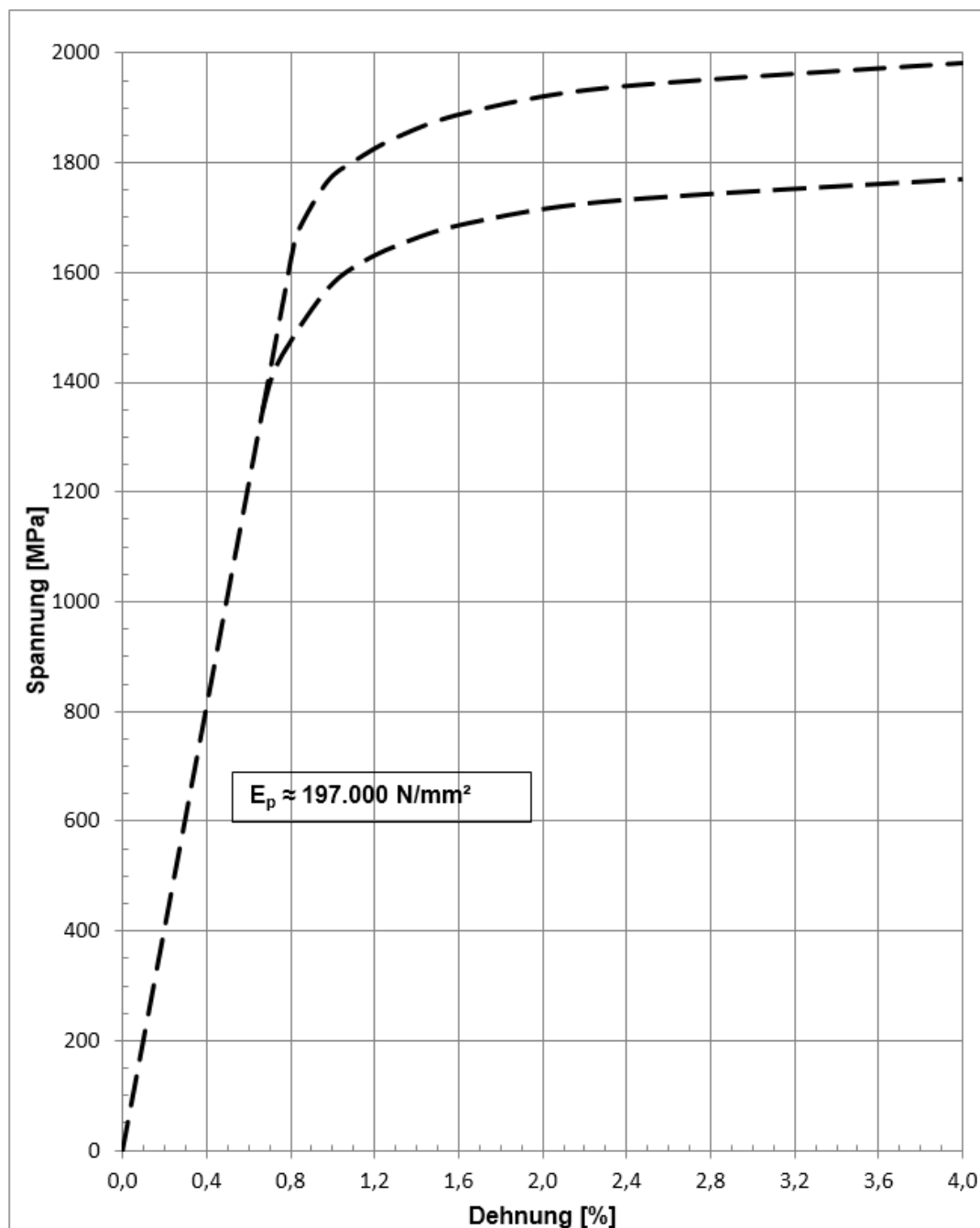
Bild 2: Prinzipieller Spannungs-Dehnungs-Verlauf
