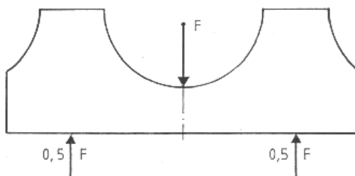
Bild 1: Belastungsanordnung Biegeversuch
