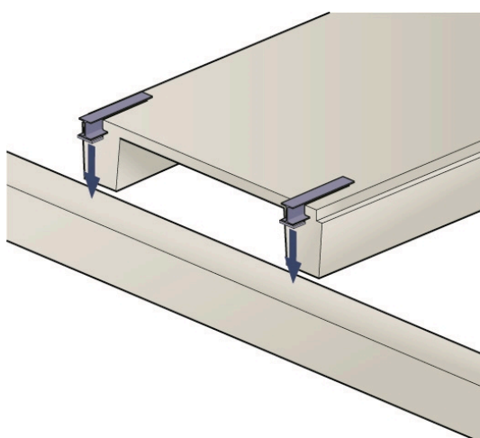
Bild 5: Trogplatten
