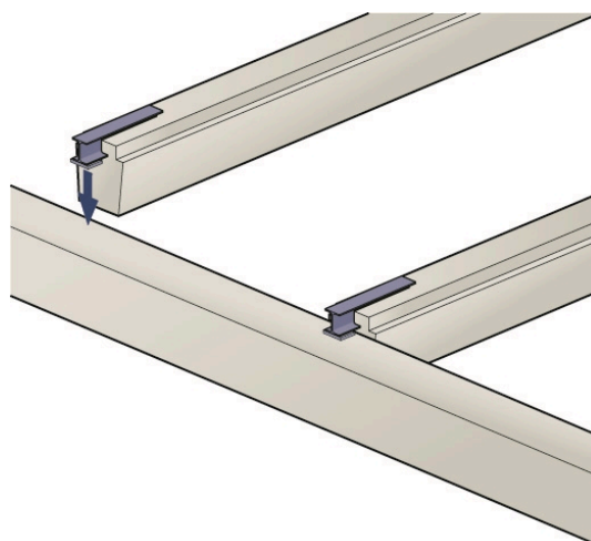
Bild 4: Nebenträger / Unterzüge
