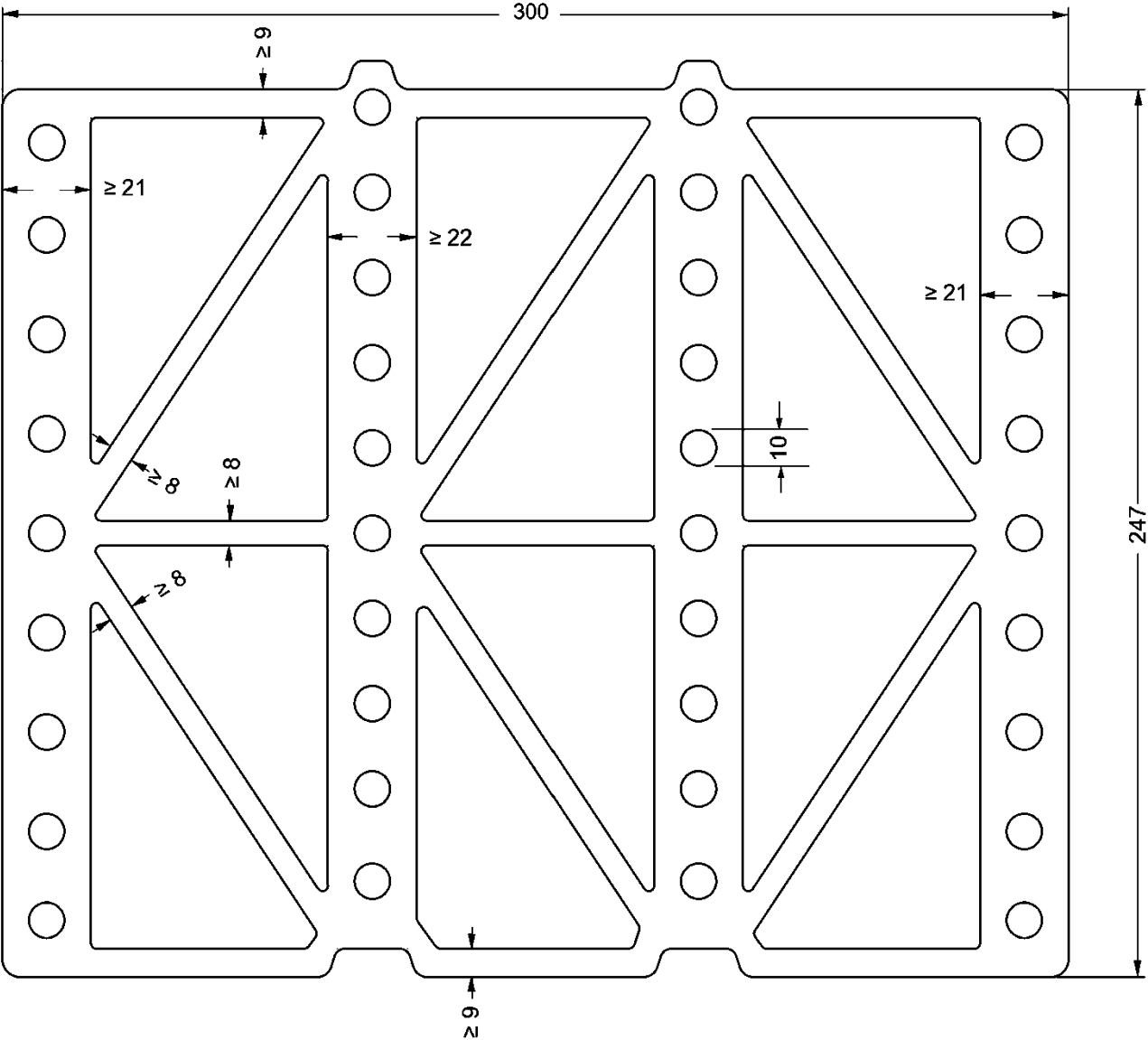
Maße in mm
