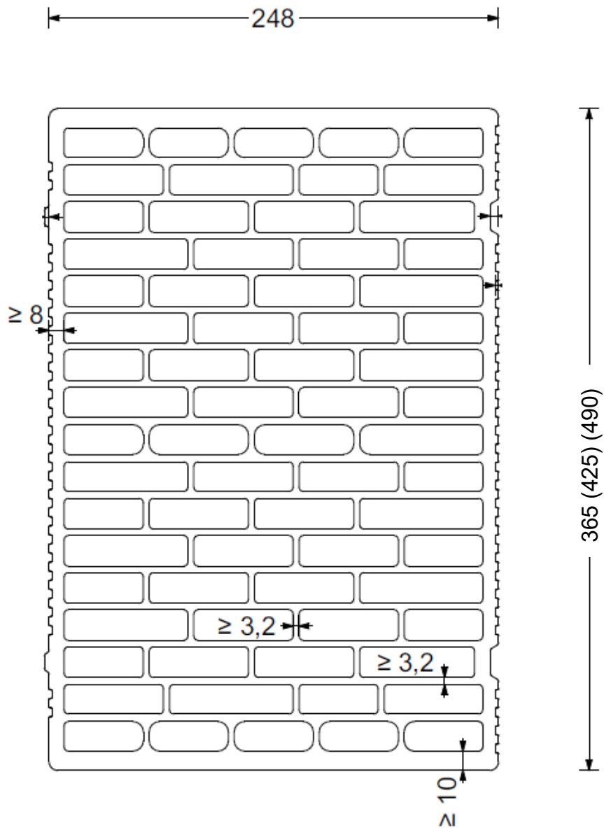
Alternative Stirnflächenausbildung unter Einhaltung der Mindeststegdicken möglich
