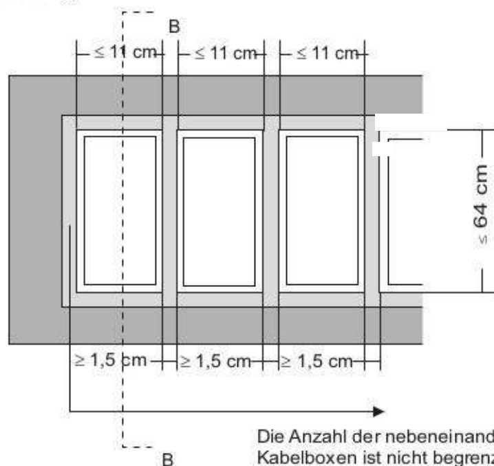
Ansicht Deckenabschottung
