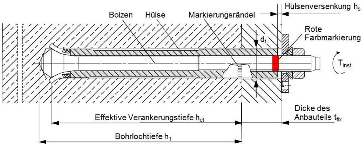
Bild 4: Durchsteckdübel HDA-T(R): Einbauzustand
