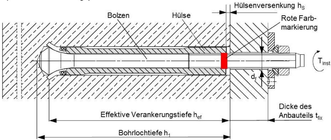
Bild 2: Vorsteckdübel HDA-P(R): Einbauzustand
