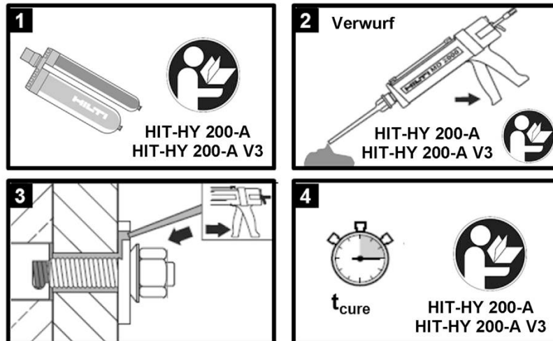
Bild 15: Montageanweisung: Verfüllung (optional) mit Injektionsmörtel Hilti HIT-HY 200-A oder Hilti HIT-HY 200-A V3
