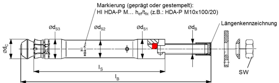
Bild 8: Vorsteckdübel HDA-P(R)
