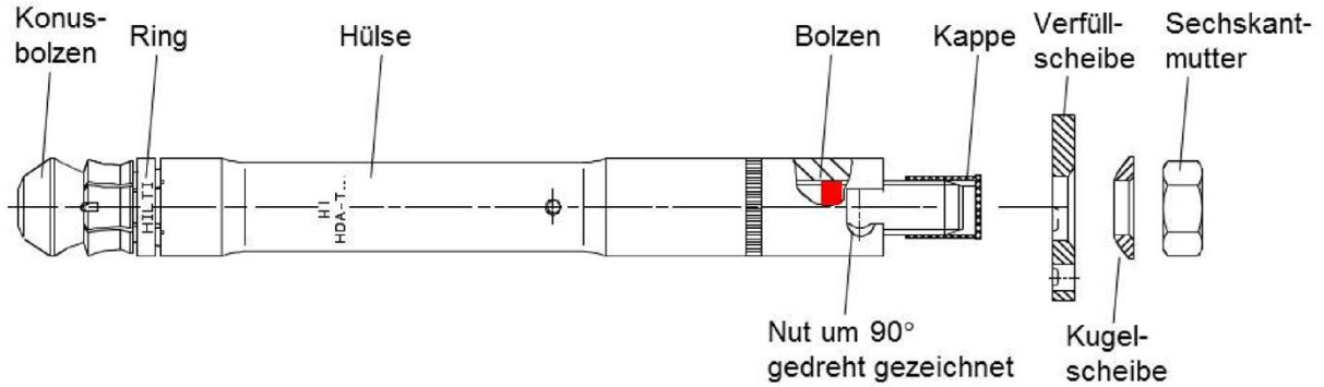
Bild 4: Durchsteckdübel HDA-T(R): Einbauzustand
