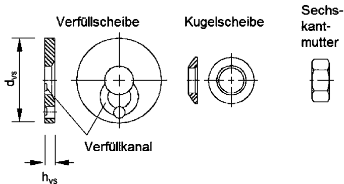
Bild 10: Verfüll-Set
