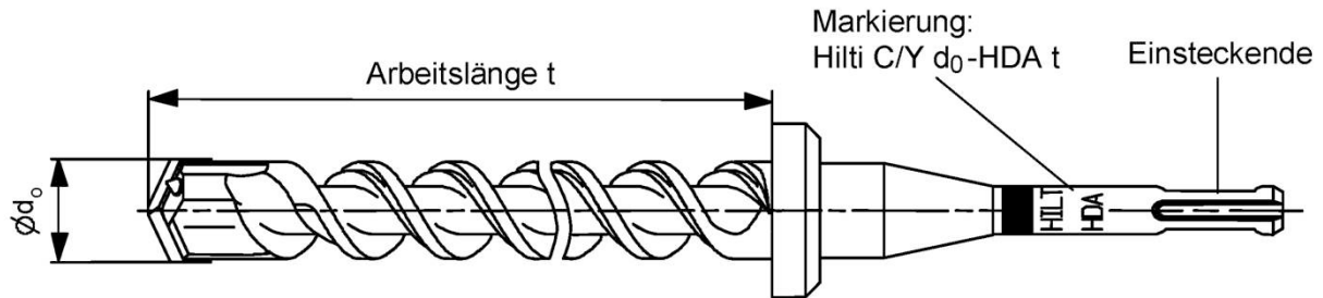
Bild 11: Bundbohrer HDA-B
