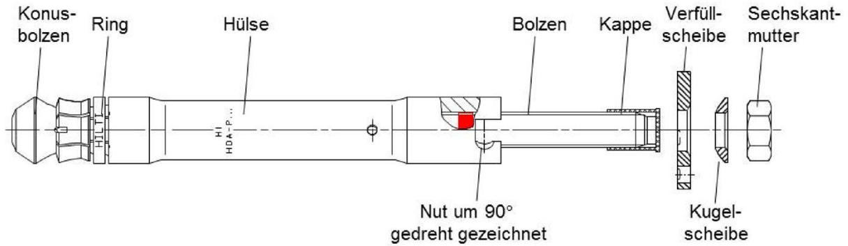
Bild 1: Vorsteckdübel HDA-P(R)
