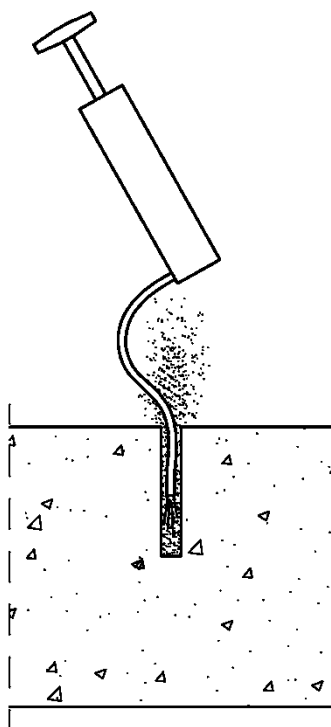
Bohrstaub entfernen
