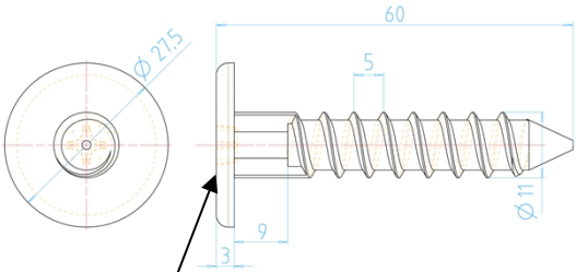
Verschlusskappe
