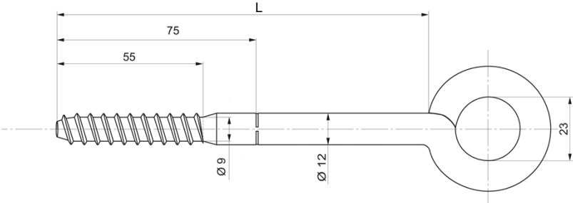
Dübel KT 14 (ETA-08/0188)
