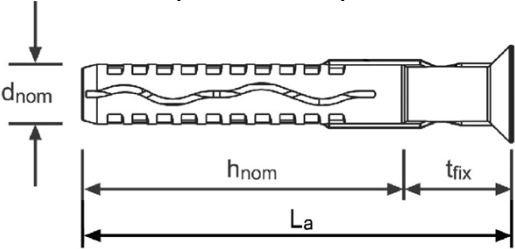
Dübel KT 14 (ETA-08/0188)
