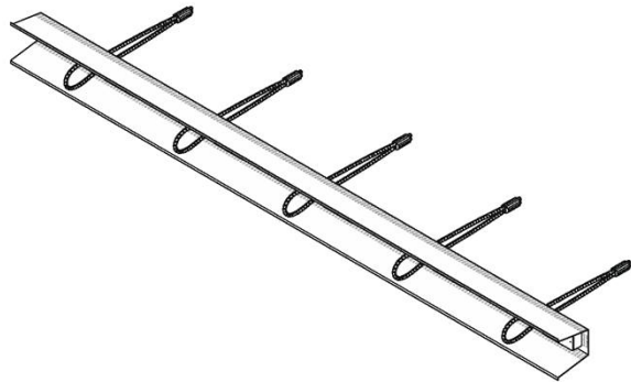
Typ 84PDS700905: tiefe Schiene
