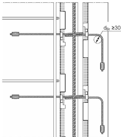
Schnitt A-A
