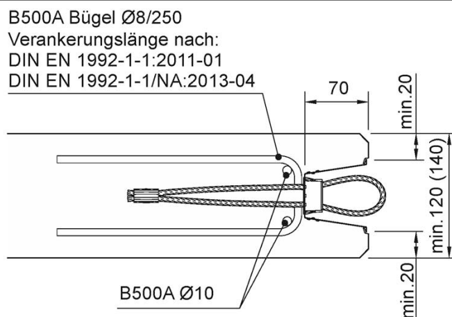
Bild 5: Bewehrung
