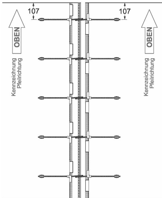
Bild 8a: Einbauvariante A Bemessungswerte gemäß Anlage 6 oder 7
