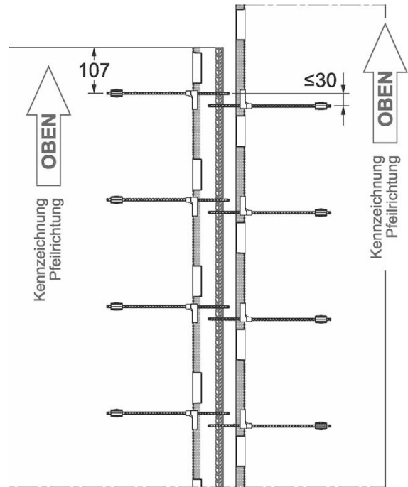
Bild 8b: Einbauvariante A Bemessungswerte gemäß Anlage 6 oder 7
