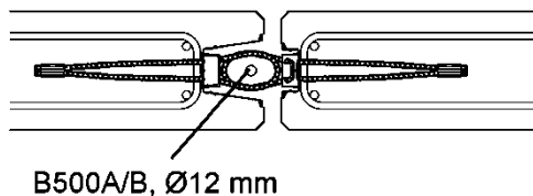
Bild 14: Anschluss Wand – Wand, Längsanschluss
