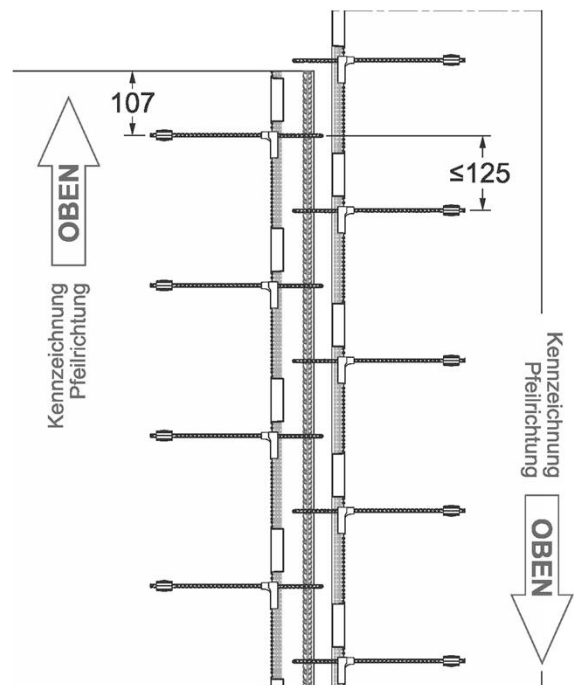
Bild 10: Einbauvariante B Bemessungswerte gemäß Anlage 8
