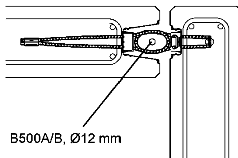
Bild 17: Anschluss Wand – Wand, Eckstoß
