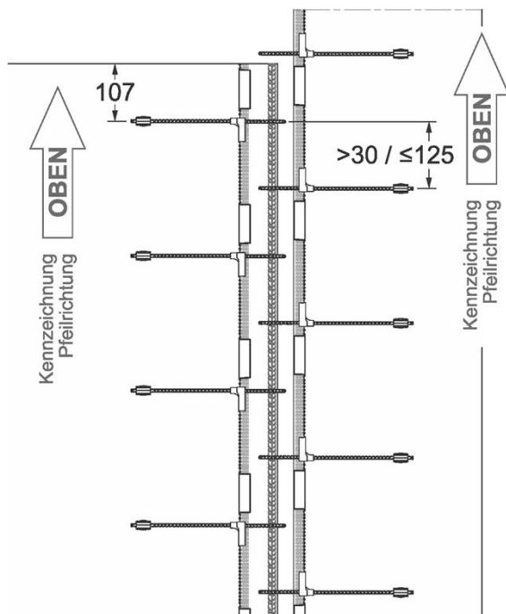
Bild 9: Einbauvariante B Bemessungswerte gemäß Anlage 8
