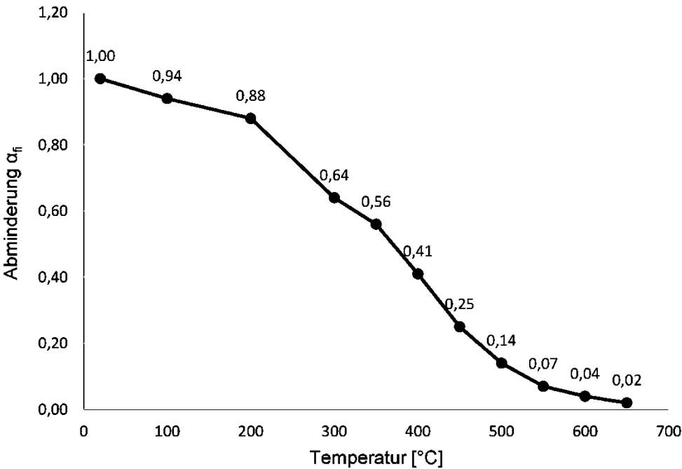
Diagramm 2: Abminderungsfaktor \alpha_{fi} in Abhängigkeit der Seiltemperatur
