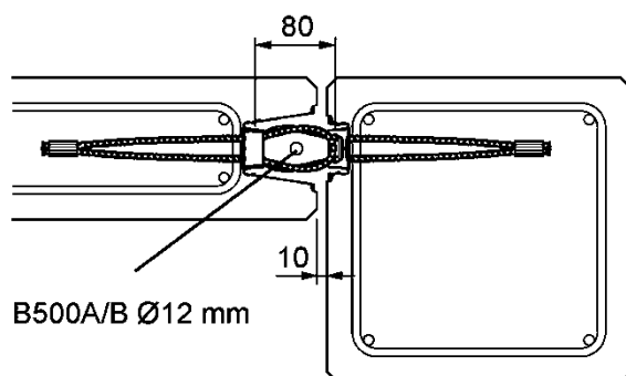
Bild 12: Minimalfuge
