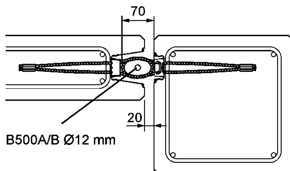
Bild 11: Horizontale Solllage
