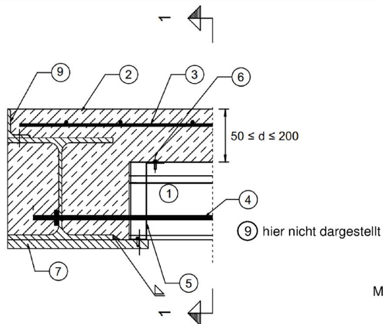
Schnitt 1-1
