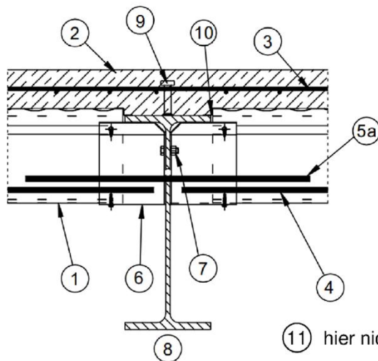
Schnitt 1-1 (5a)
