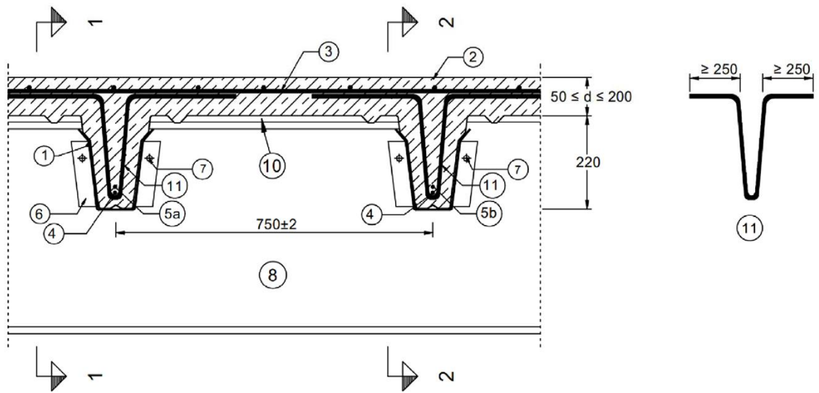
Schnitt 1-1 (5a)
