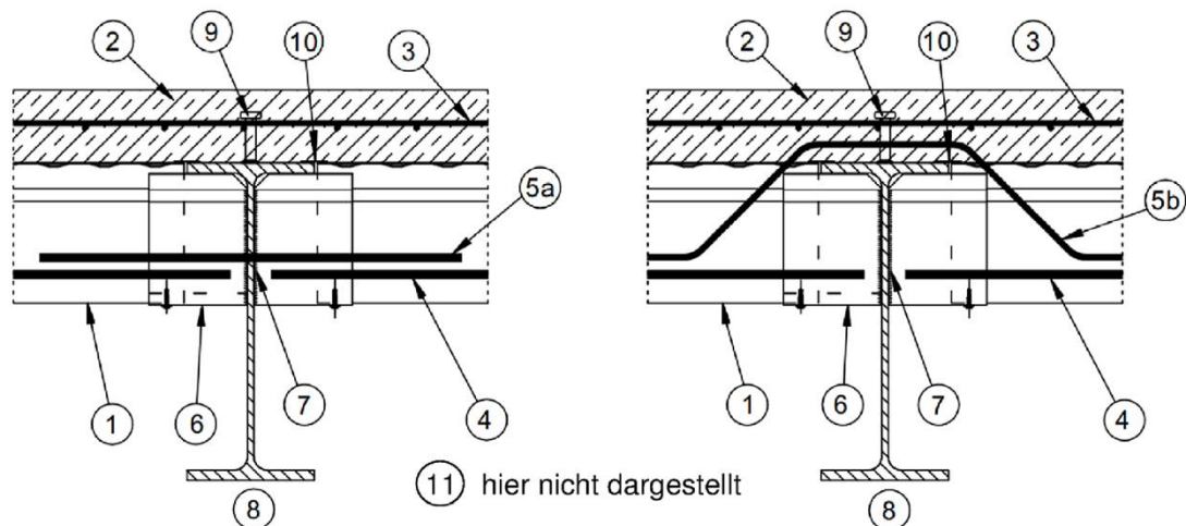
Schnitt 1-1 (5a)
