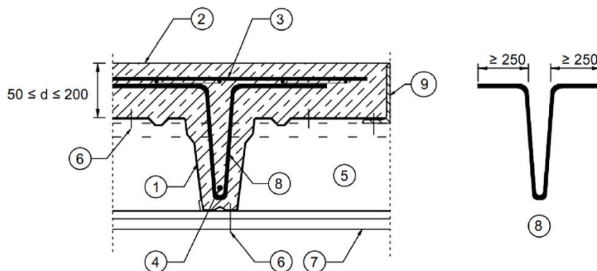
Schnitt 1-1
