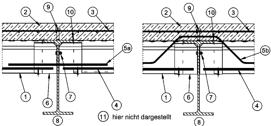
Schnitt 1-1 (5a)
