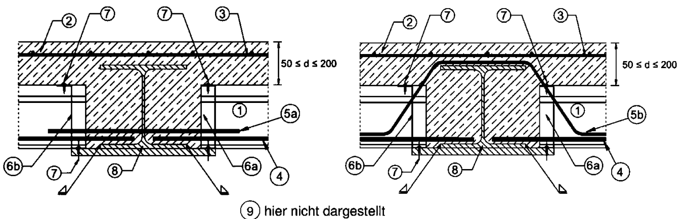
Schnitt 2-2 (5b)
