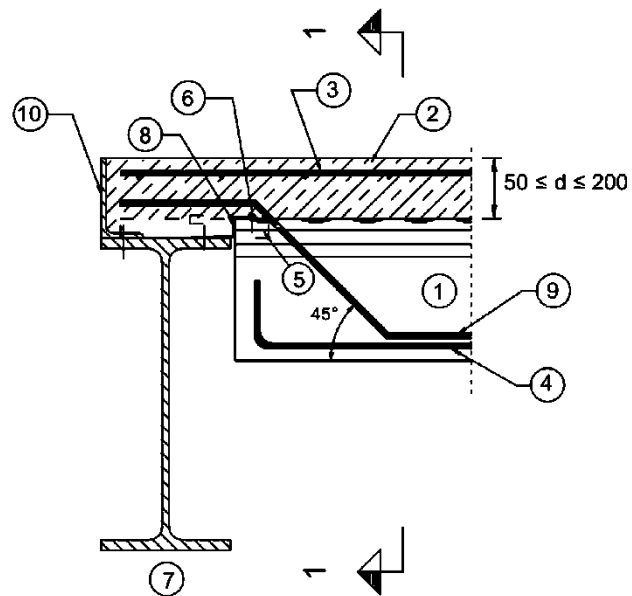
Schnitt 1-1
