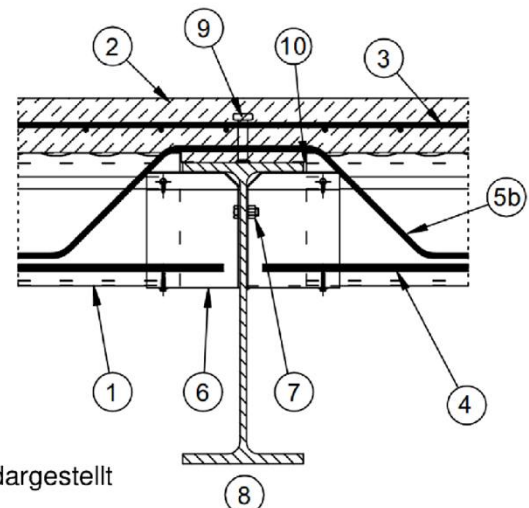
Schnitt 2-2 (5b)
