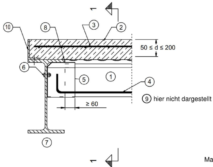
Schnitt 1-1
