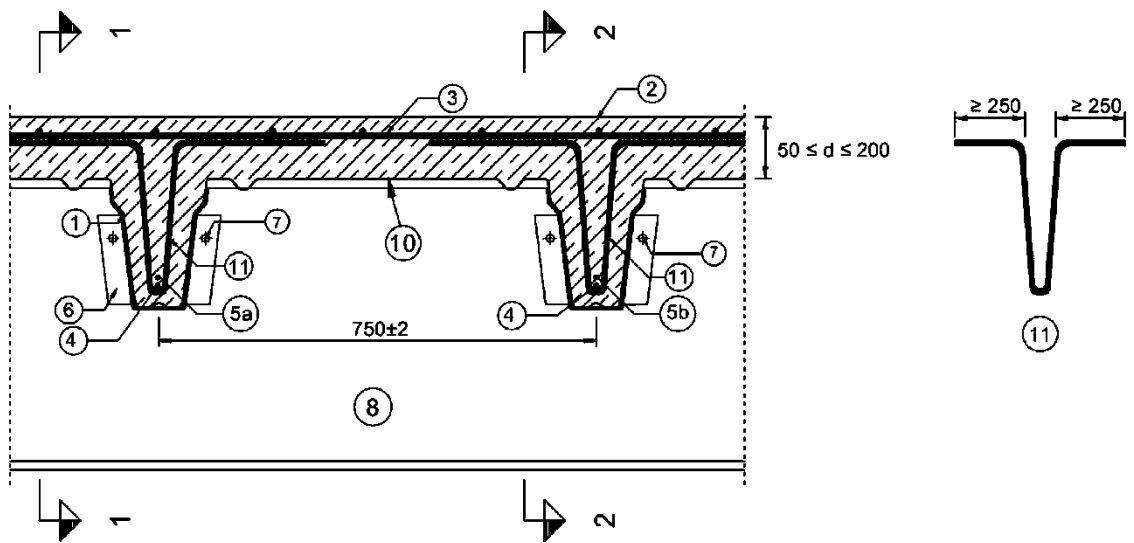
Schnitt 1-1 (5a)
