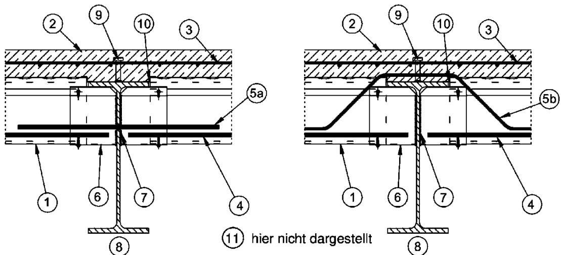
Schnitt 1-1 (5a)
