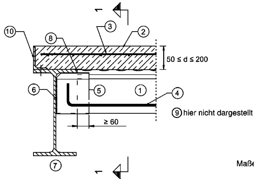
Schnitt 1-1
