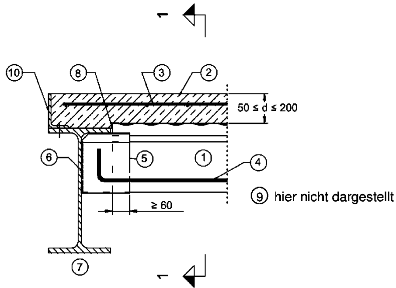
Schnitt 1-1
