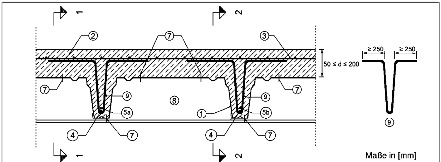
Schnitt 1-1 (5a)
