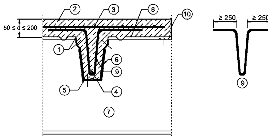
Schnitt 1-1
