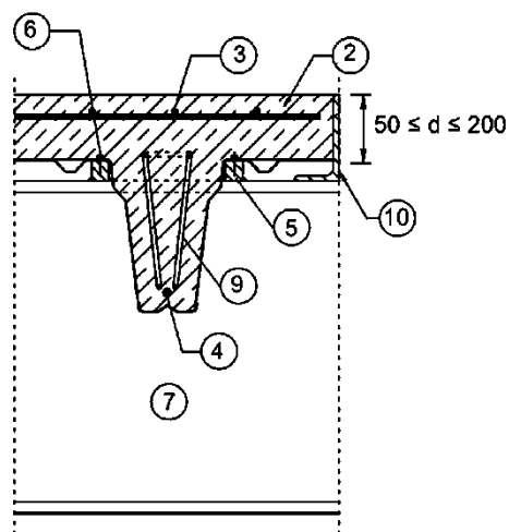
Schnitt 1-1
