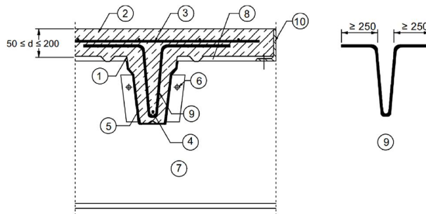
Schnitt 1-1
