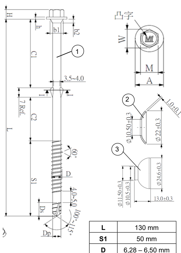
Bild 2.10: Shen Fung Spezialbohrschraube 6,5 x 130 mm für Holz-Unterkonstruktion
