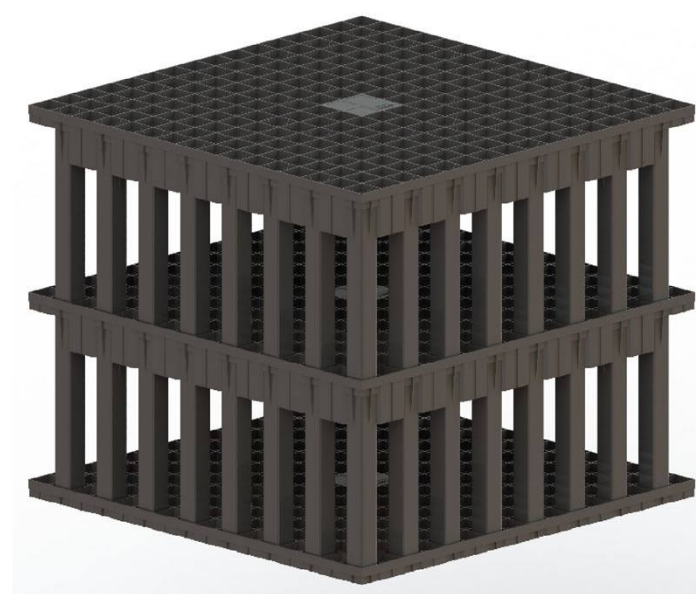
Aufbau 2-lagig (1 x Bodenplatte und 2 x Grundelement)
