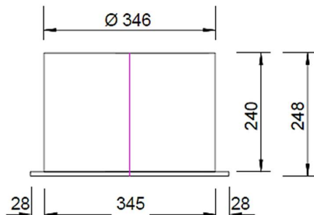
Ansicht vorne/hinten
