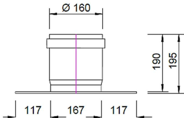
Ansicht vorne/hinten
