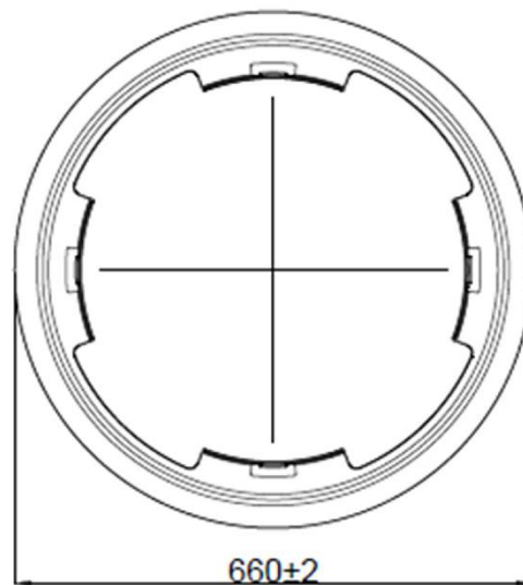
Draufsicht:
