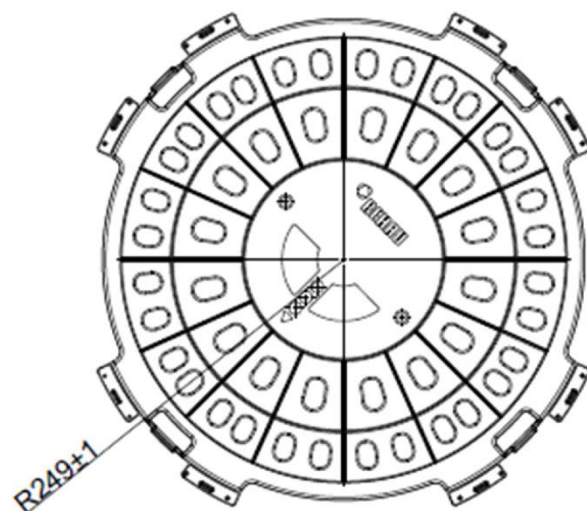
Draufsicht:
