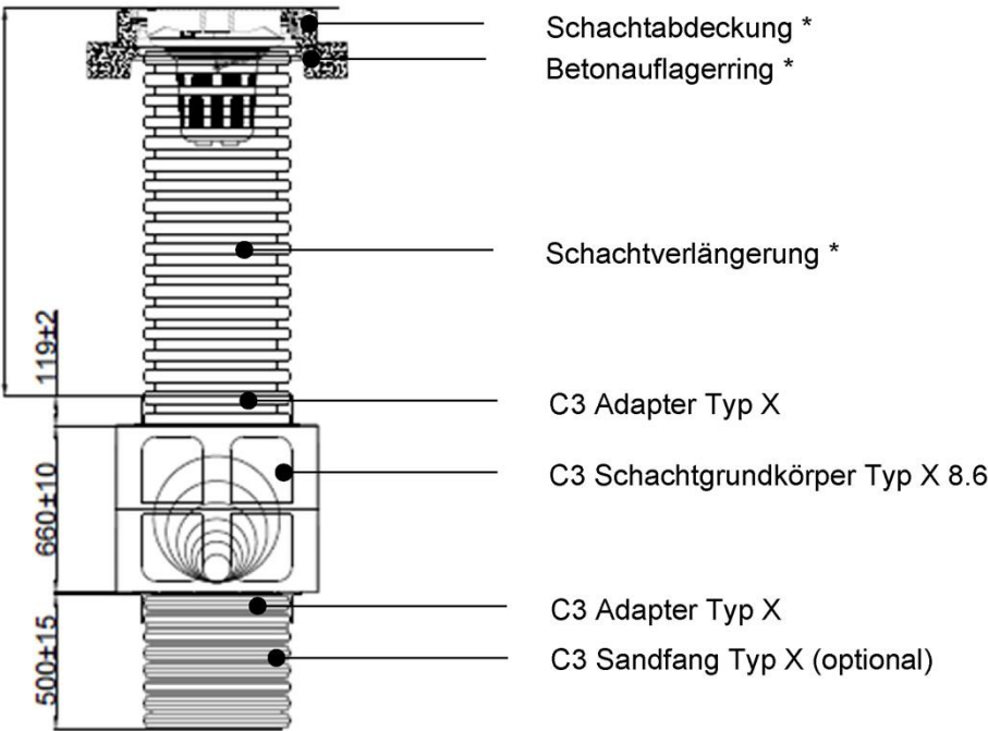
2 ½-lagiger Aufbau C3-Schacht Typ X:
