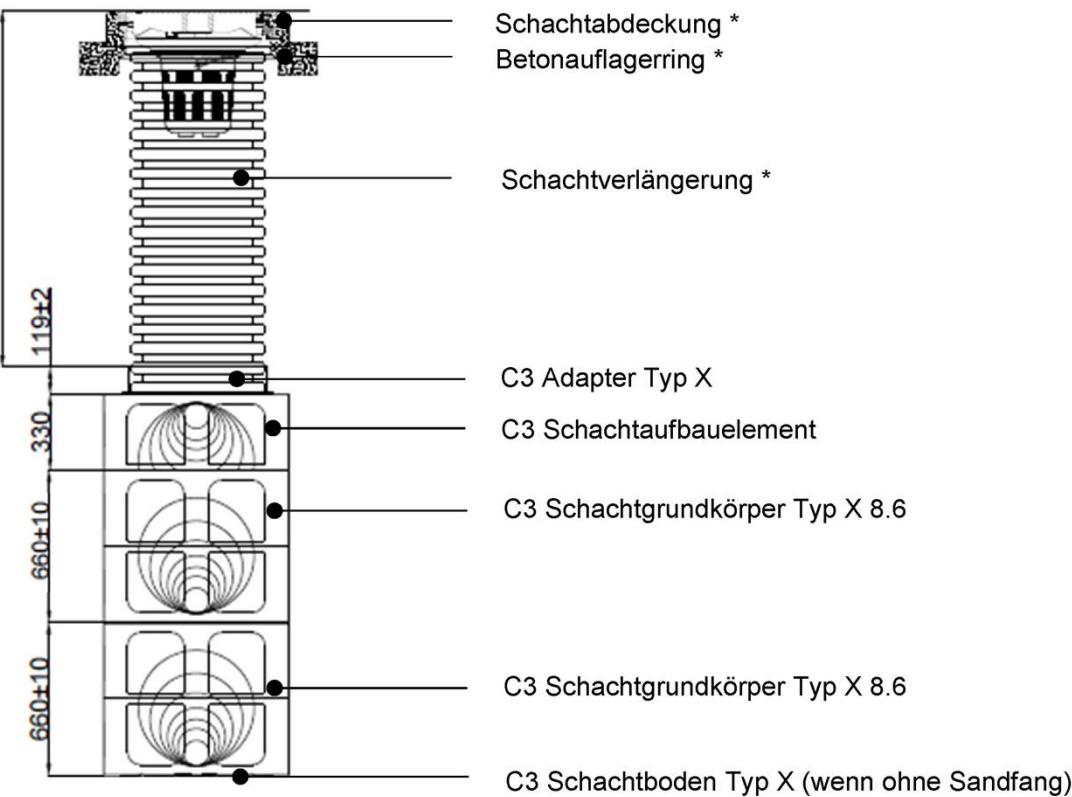
2 ½-lagiger Aufbau C3-Schacht Typ X:
