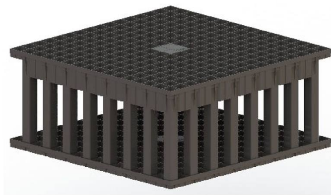
Aufbau 1-lagig (1 x Bodenplatte und 1 x Grundelement)
