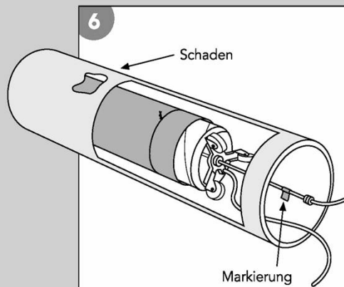
Packer an Schadstelle vorschieben und gemäß Markierung Schiebestange positionieren
