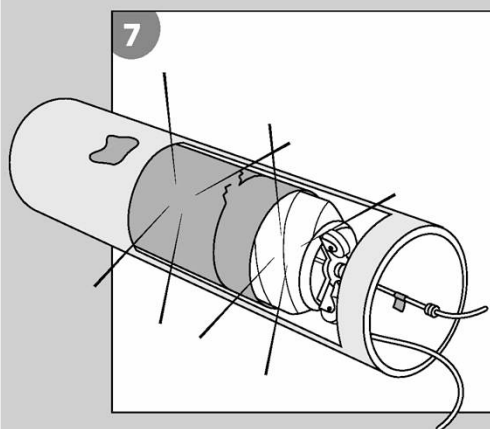
Packer an der Schadstelle mit vorgeschriebenen Druck anblasen und LED- Licht einschalten
