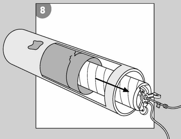
Nach Ablauf der Aushärtezeit LED-Licht ausschalten und nach Wartezeit Druck ablassen und Packer aus Rohrleitung entfernen
