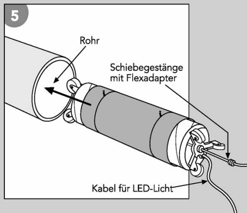
Schiebestange und Flexadapter an Luftanschluss des Packers befestigen. Sicherungsseil anbringen
