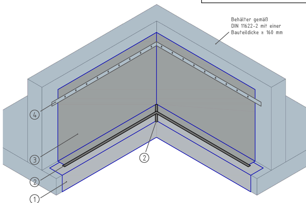
Abbildung 2: Ausführung Innenecke
