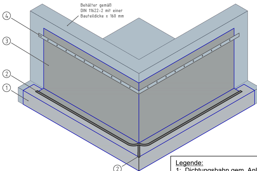
Abbildung 1: Ausführung Außenecke
