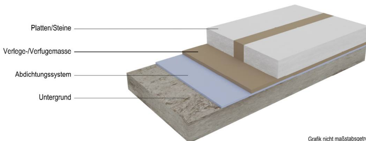
Abbildung 1: Kombiniertes Auskleidungssystem mit Beschichtungssystem und Nutzschicht aus Platten oder Steinen gemäß Tabelle 1 verfugt mit Kunstharzkitt Stellagen VEQ
