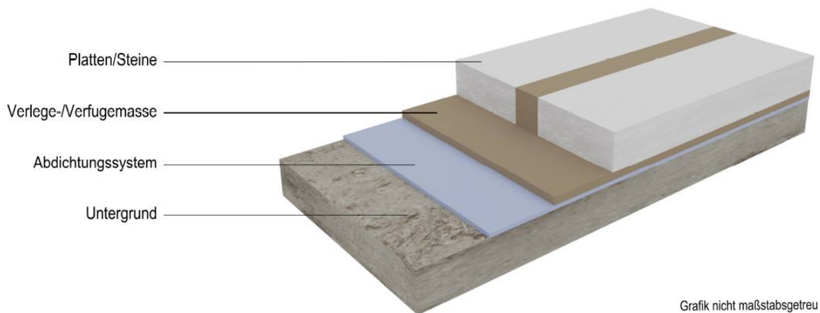
Abbildung 1: Systemaufbau Stellagen SC CM 1 (nicht ableitfähig) mit Abdichtungssystem Stellagen SC-GF AS (Beschichtungssystemvarianten 1 und 2) und Kittsystem Stellagen SC Kitt
