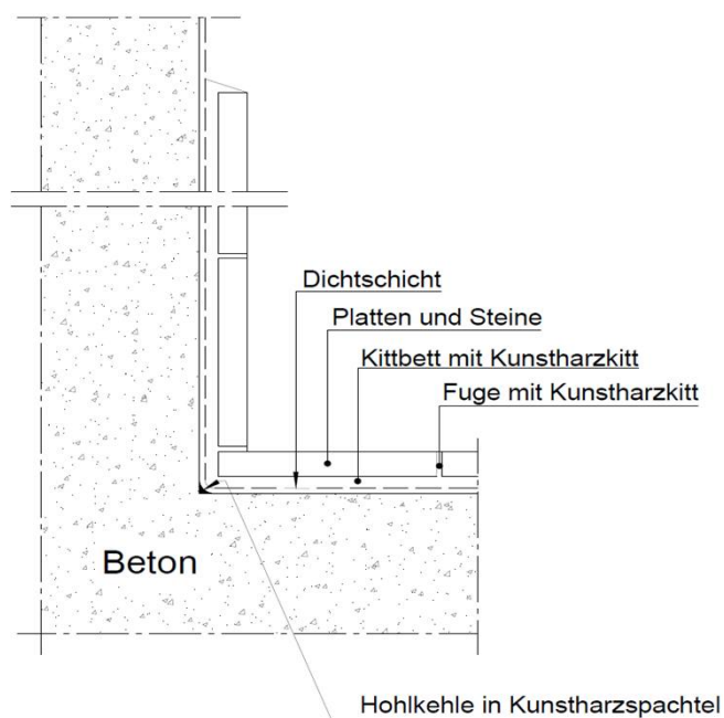
Abbildung 1: Boden-/Wandanschluss und Sockelausbildung
