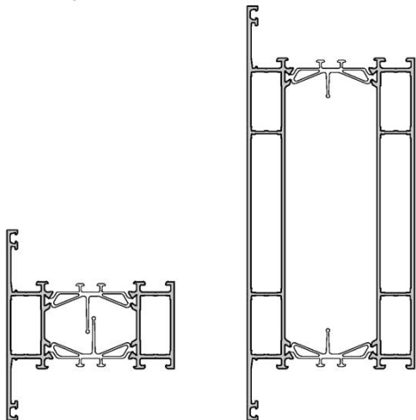
Darstellungen M1:3
