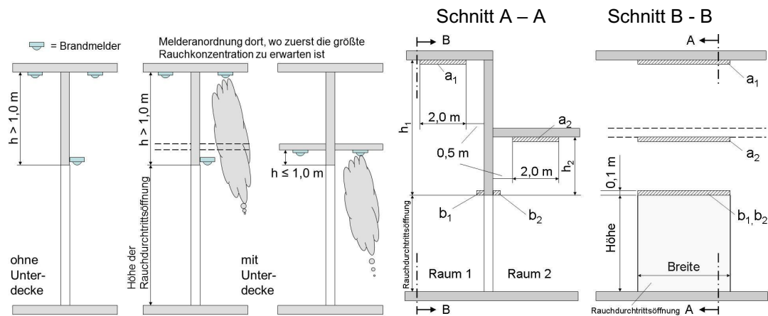
Bild 2: Maßgebende Höhe der Deckenunterfläche Bild 3: Installationsbereiche
