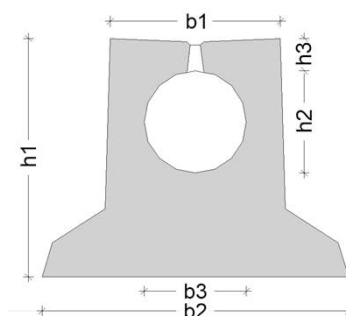
Querschnittsvariante 3 (FU)
