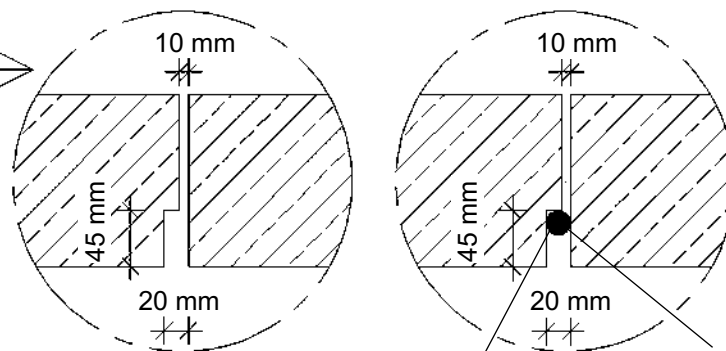
Detail Verbindungsfuge
