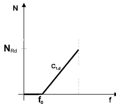
Bild 3: Bilineare Steifigkeit
