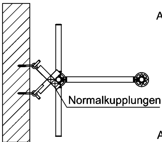
Gerüstlage ohne Konsole
