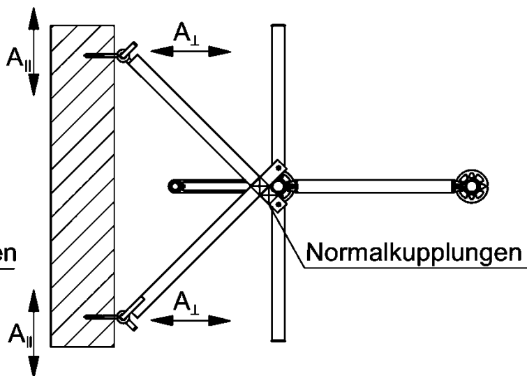
Gerüstlage mit Konsole
