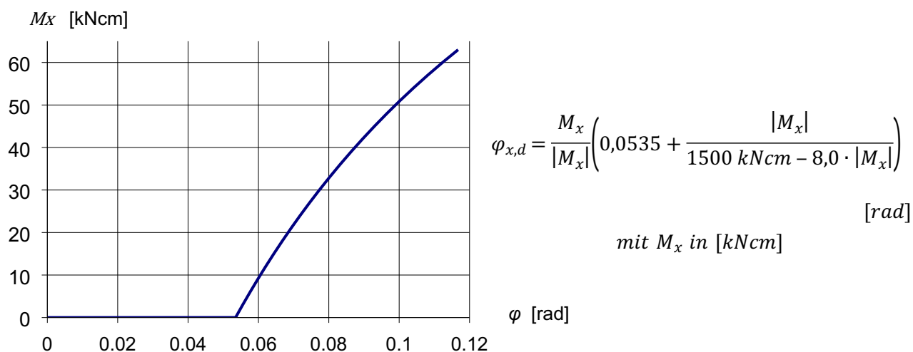
Bild A4: Drehfedersteifigkeit im O-Riegelanschluss bei Torsion um die Riegelachse
