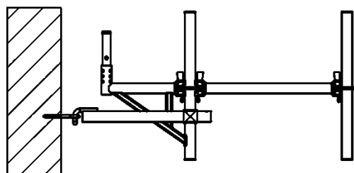
Gerüstlage mit Konsole
