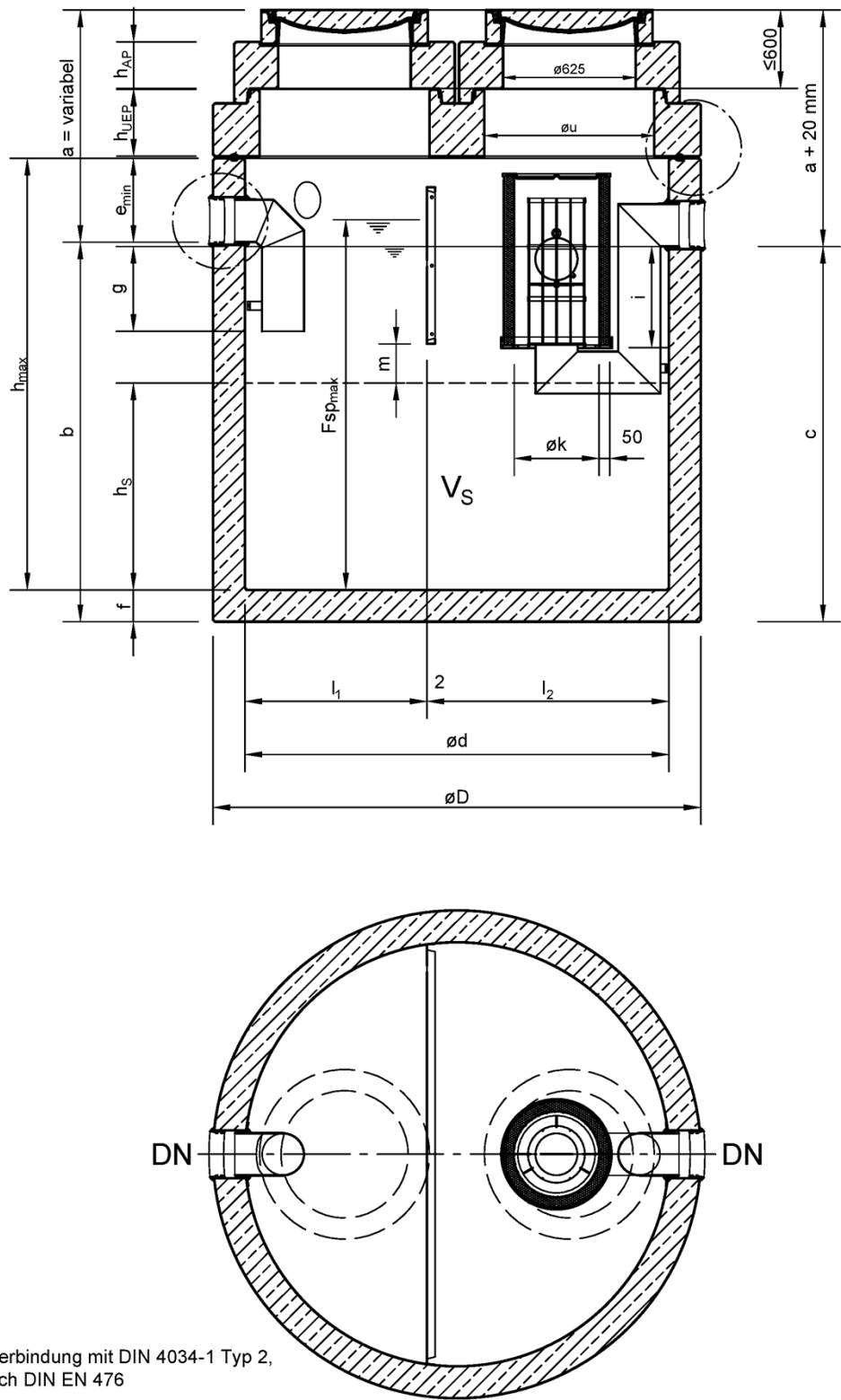
Sedimentations- und Abscheideeinrichtung NeutraPro
