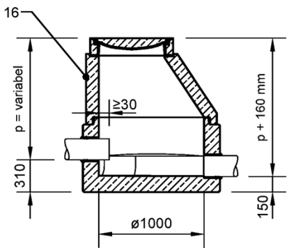
Probenahmeschacht
