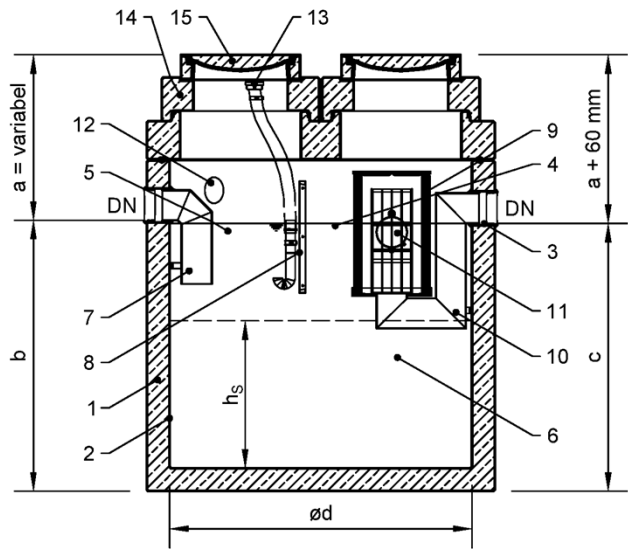
Sedimentations-/ und Abscheideeinrichtung NeutraPro
