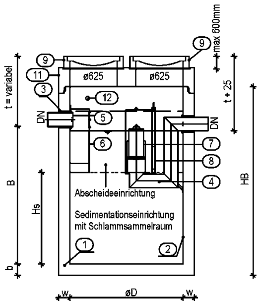
Abscheideeinrichtung Typ Ekotek KA-I mit Koaleszenzeinrichtung
