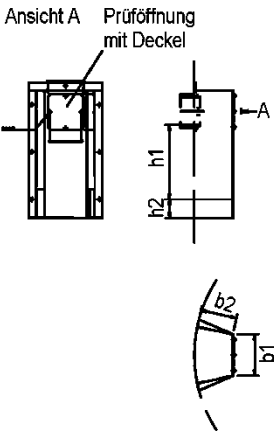
Detail Zulaufkasten
