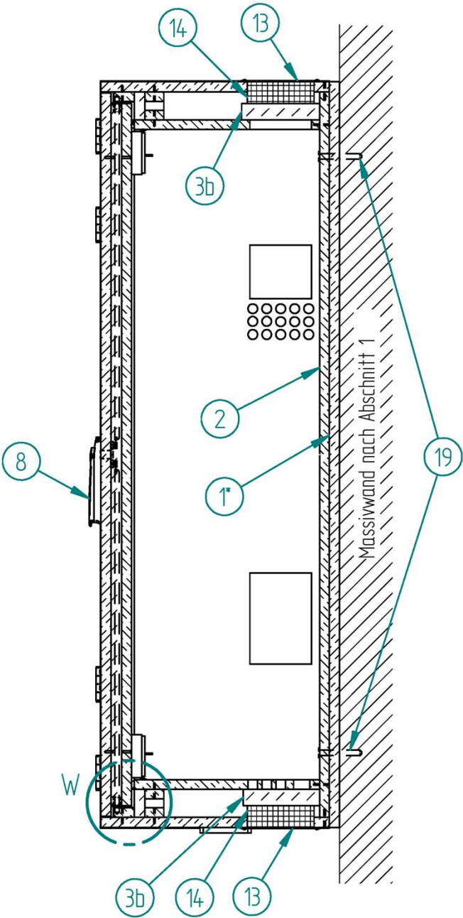
Schnitt D-D
