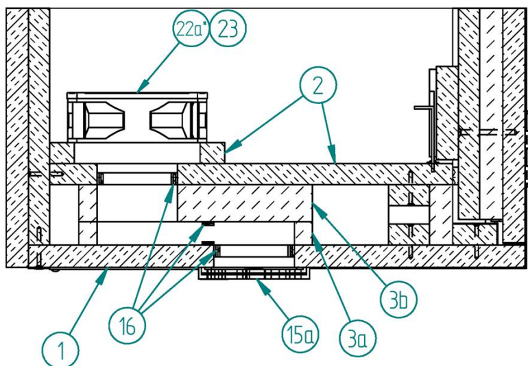
Schnitt E-E
