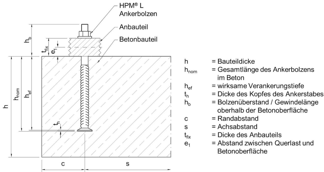
Abbildung 1: Allgemeine Montage
