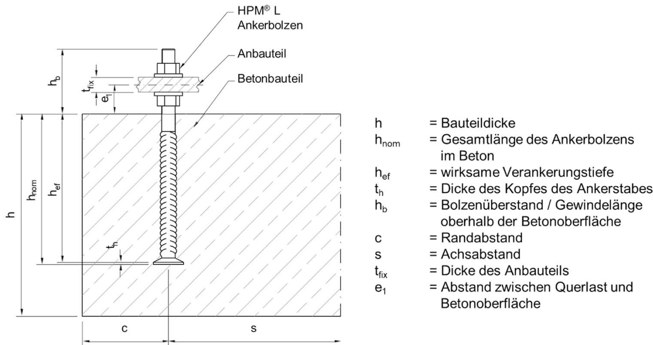
Abbildung 2: Stahl-Stahl-Kontakt (Abstandsmontage)
