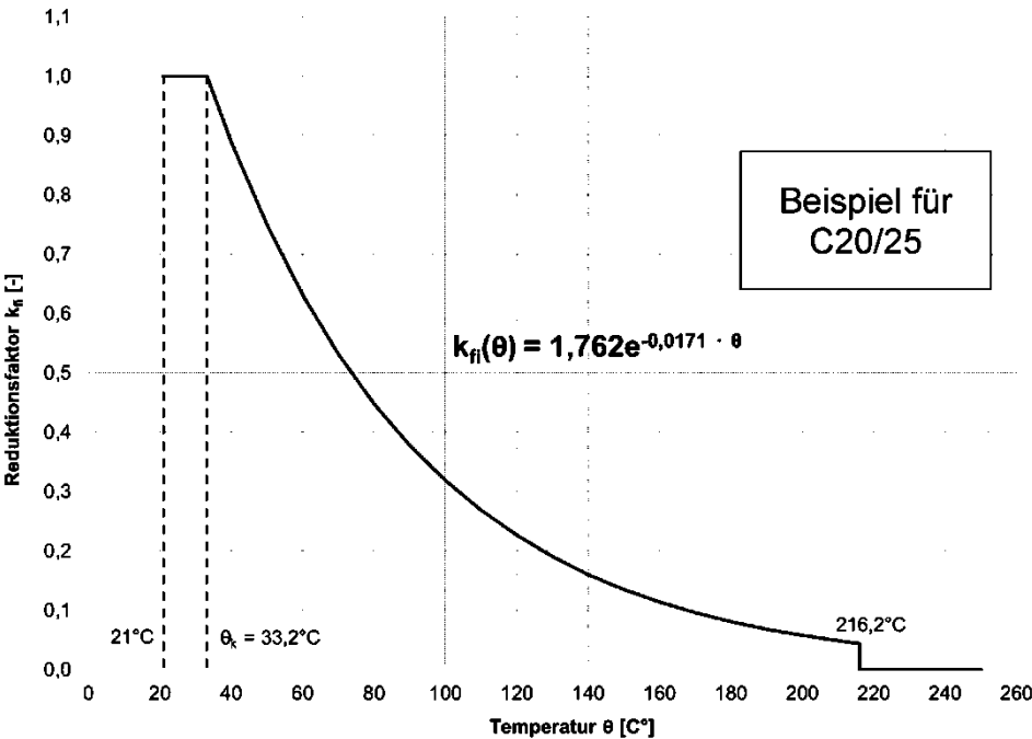
Bild C1 Beispieldiagramm des Temperaturabminderungsfaktors k_{fi}(\theta) = k_{fi,100y}(\theta) für Betonfestigkeitsklasse C20/25 bei guten Verbundbedingungen:
