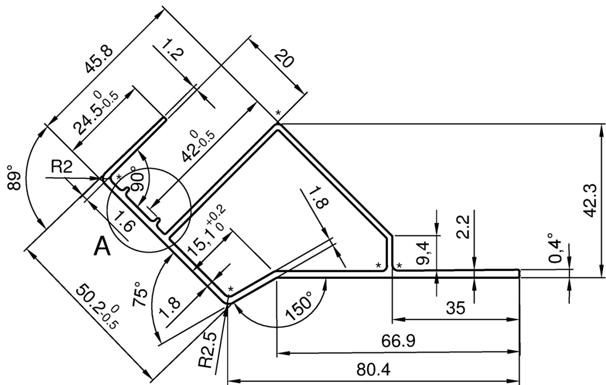
Auflagerprofil 3
