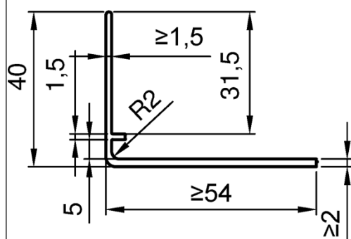
Abdeckwinkel
