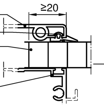
Schnitt A-A (alternativ)
