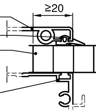
Schnitt A-A (alternativ)
