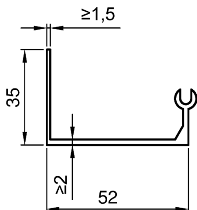
Randprofil
