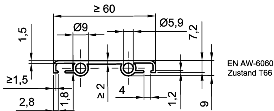
Abdeckprofil 2
