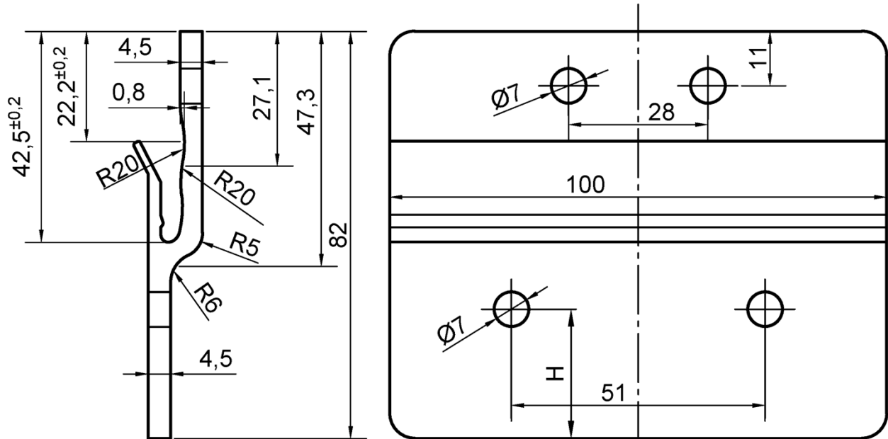
Spannkonsole 2
