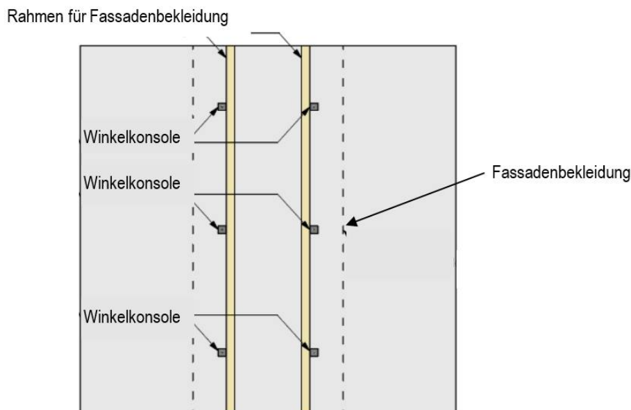
Bild B1.2: Beispiel einer statisch unbestimmten Befestigung für die Verankerung von Fassadenbekleidungen
