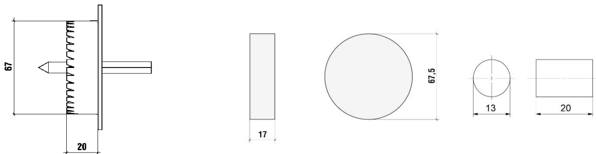
Setzwerkzeug WK-FT/WK-FM für die tiefgesetzte Montage
