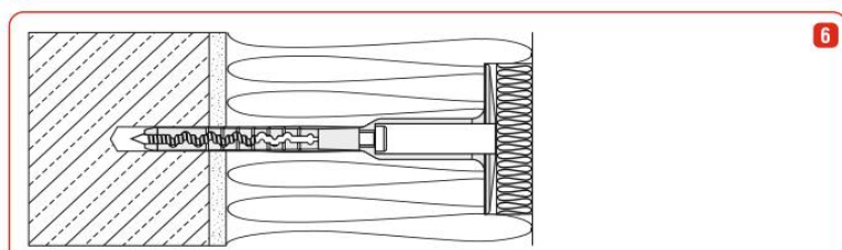
Abb. 6 Einbauzustand.
