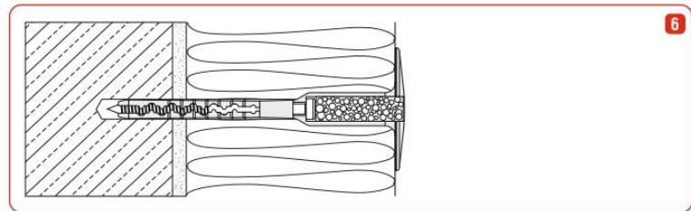
Abb. 6 Eingebauter Zustand.
