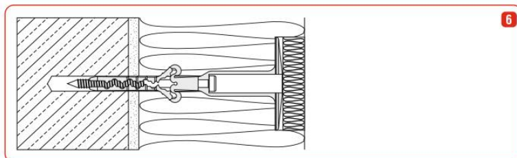
Abb. 6 Einbauzustand.
