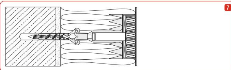
Abb. 7 Eingebauter Zustand.
