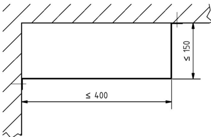
2-seitiger Installationskanal
