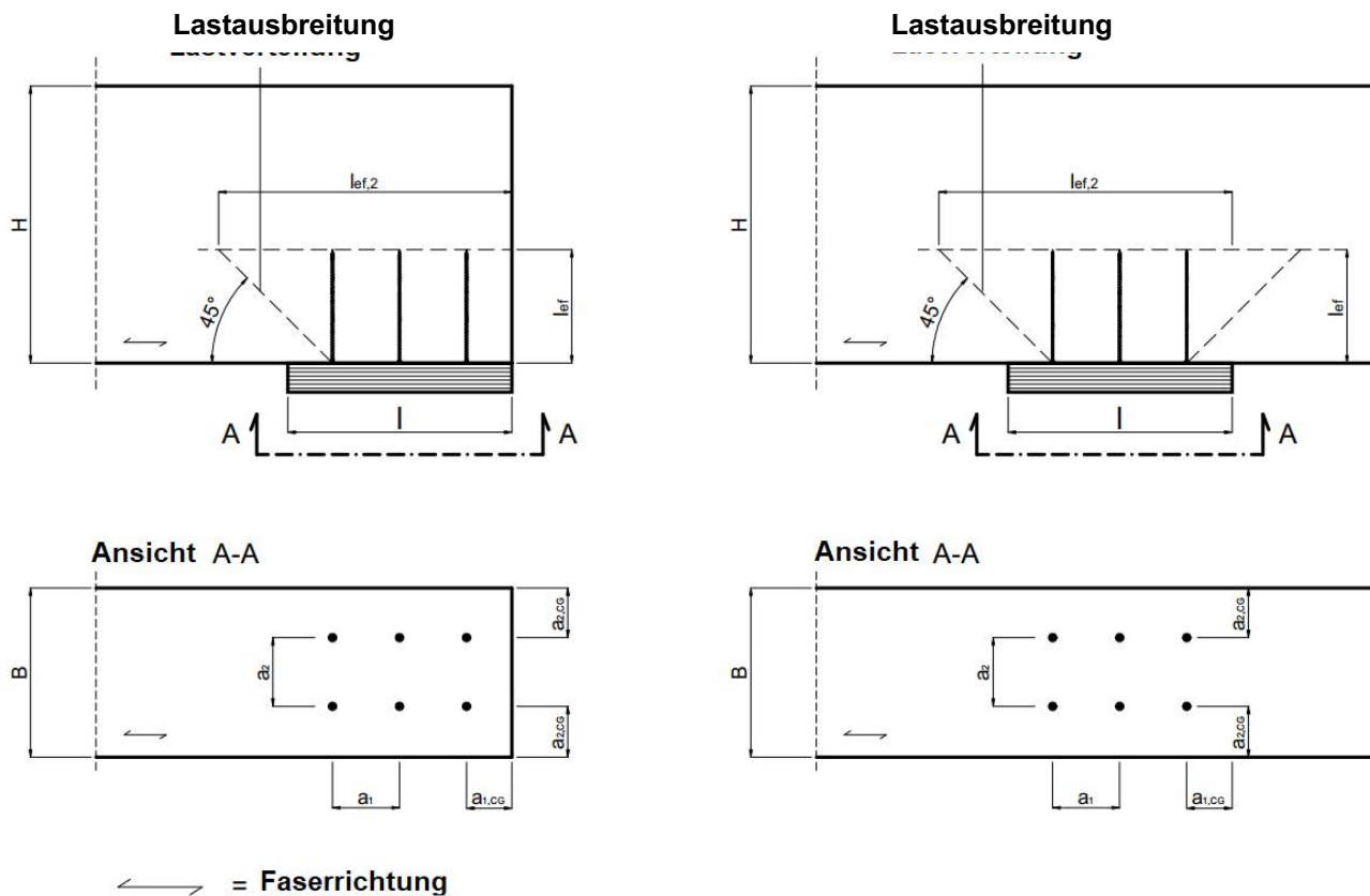
Abbildung A.3.1 Verstärktes Endauflager (links) und verstärktes Zwischenauflager (rechts)
