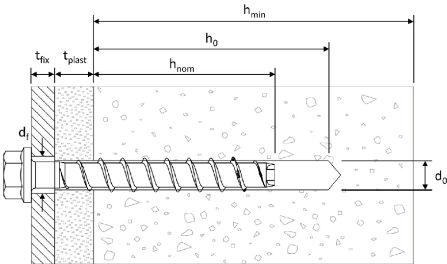
PERMALAST Betonschraube SCREW BOLT-1000 LT im Vollbaustoff und Lochbaustoff mit nichttragender Schicht
