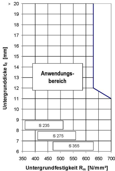
Baustahl nach EN 10025-2
