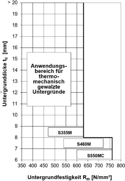
Baustahl nach EN 10025-4 und EN 10149-2
