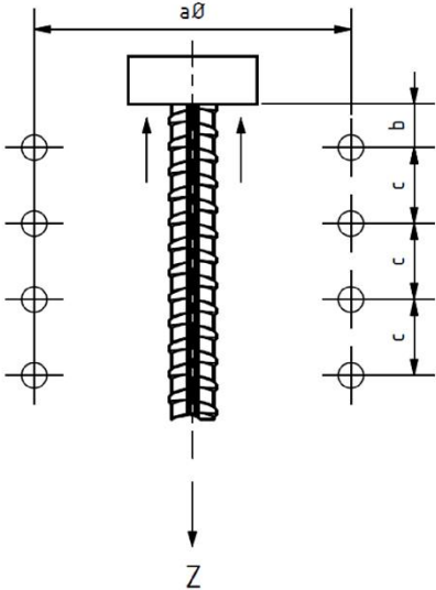
Bei Zugbeanspruchung
