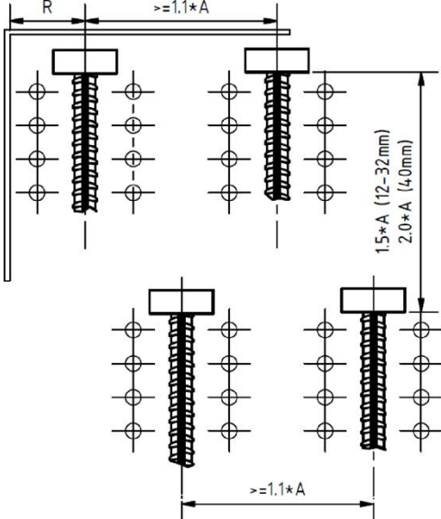
Versetzte Verankerung
