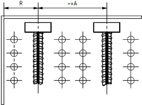
Unversetzte Verankerung
