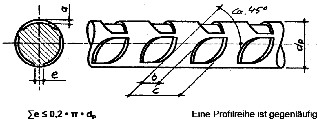
Bild 1: Ansicht des sonderprofilierten Spannstahls
