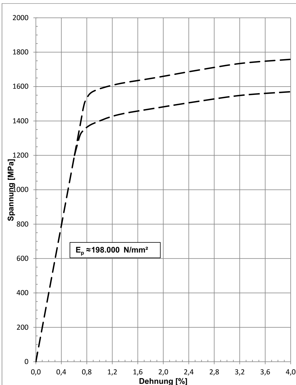
Bild 2: Prinzipieller Spannungs-Dehnungs-Verlauf
