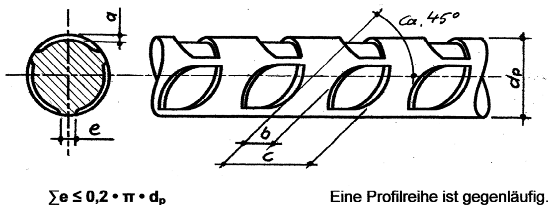
Bild 1: Ansicht des sonderprofilierten Spannstahls
