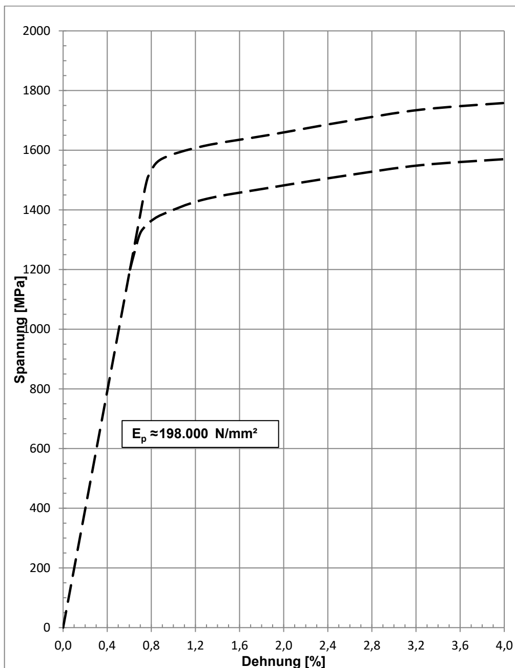
Bild 2: Prinzipieller Spannungs-Dehnungs-Verlauf
