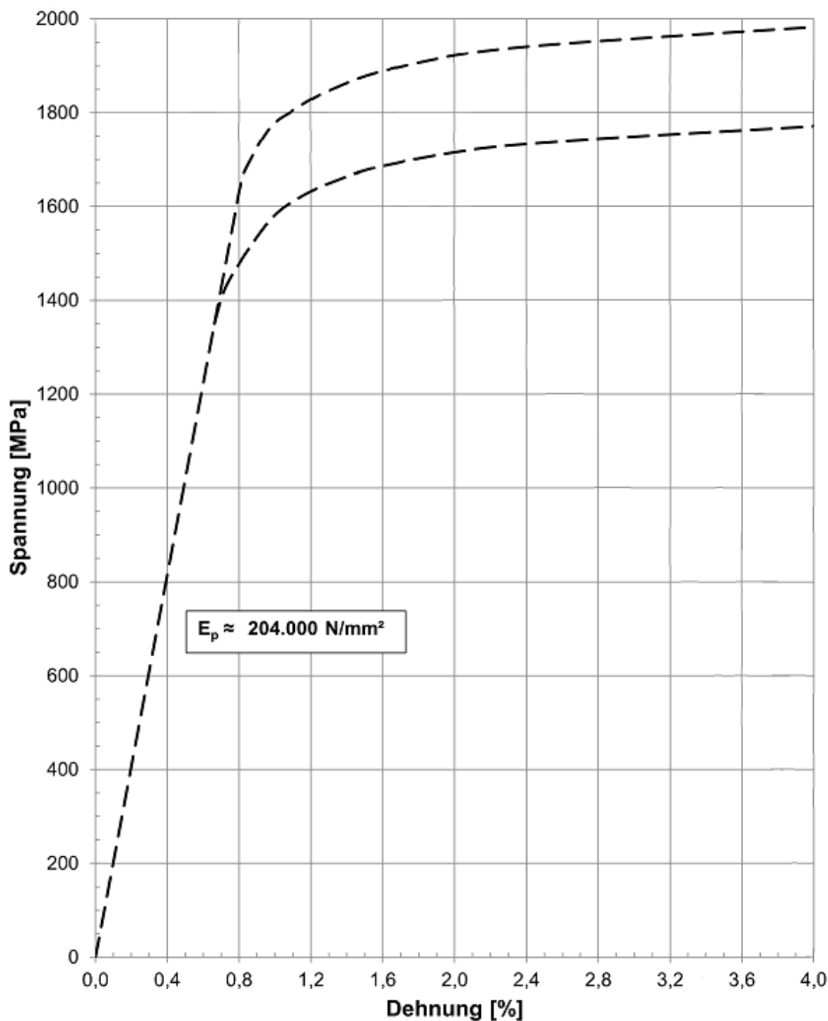
Bild 2: Prinzipieller Spannungs-Dehnungs-Verlauf
