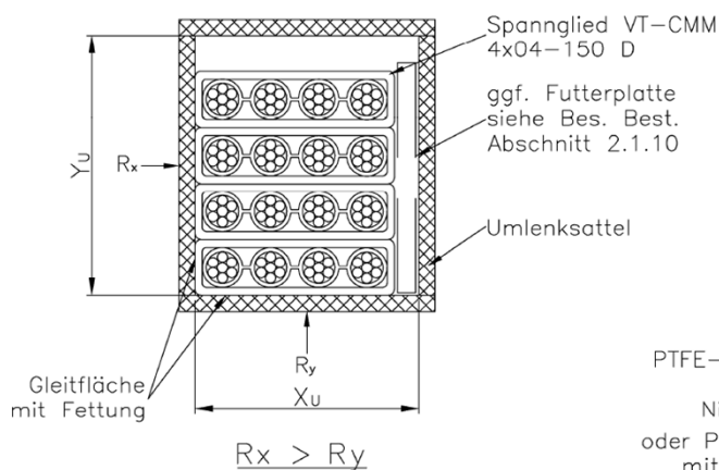
Schnitt A-A (Umlenksattel Kunststoff)
