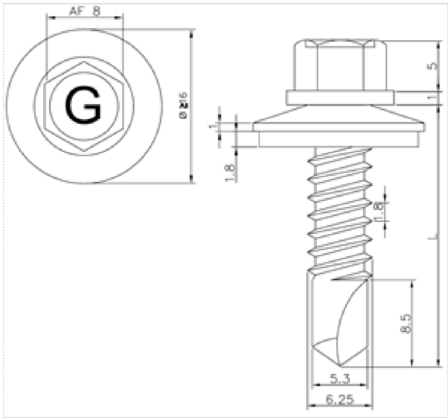
Bohrschraube GO-BOHR 6.3x25
